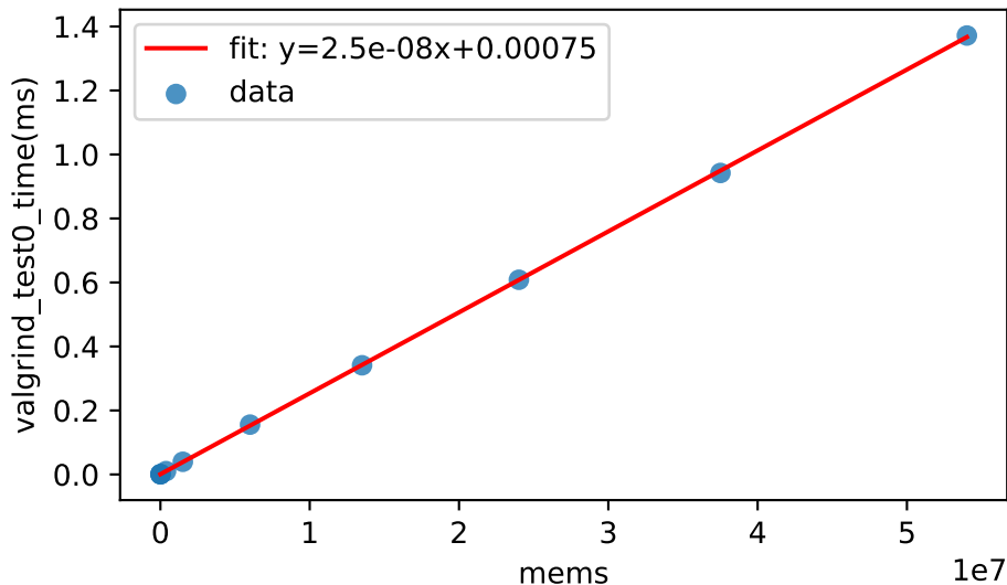
insertsort: mems vs. valgrind_test0_time(ms) Pearson r=1.000 , R^2=1.000
