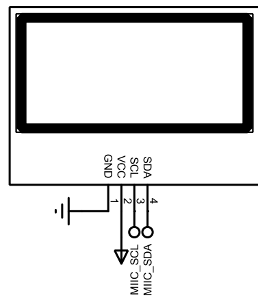
LCD1 OLED12864I2C
