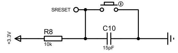
复位电路
