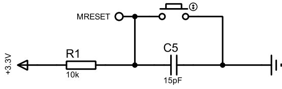
复位电路
