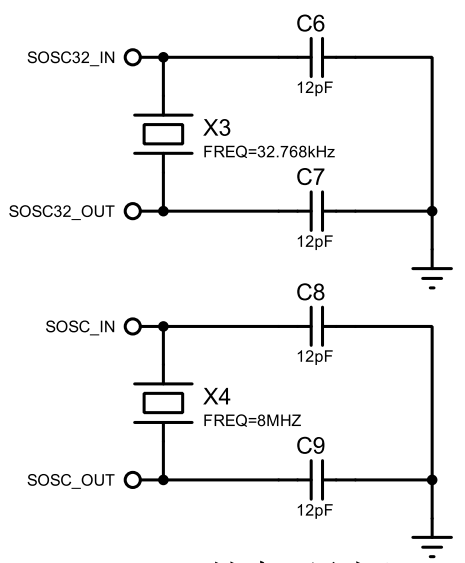
从机晶振
