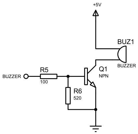
蜂鸣器
