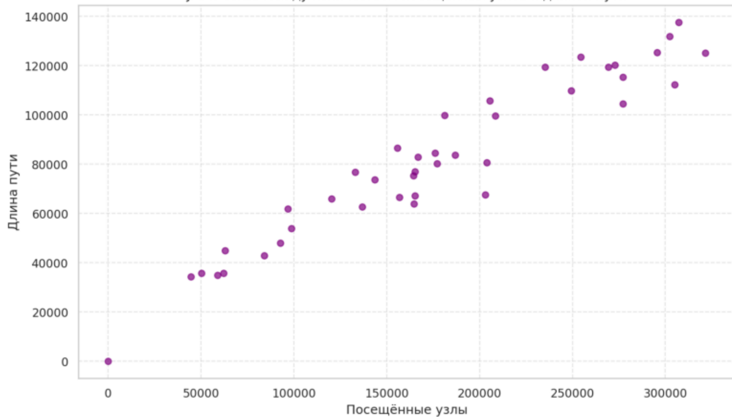
JPS4: Связь между количеством посещённых узлов и длиной пути
