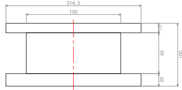
主视图 FRONT VIEW
