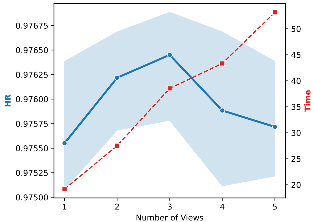
Dataset: VID
