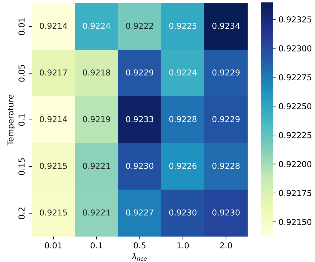
Dataset: VID
