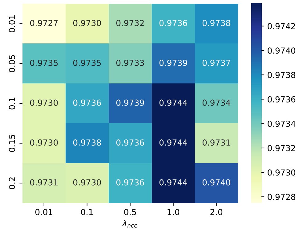
Dataset: VID
