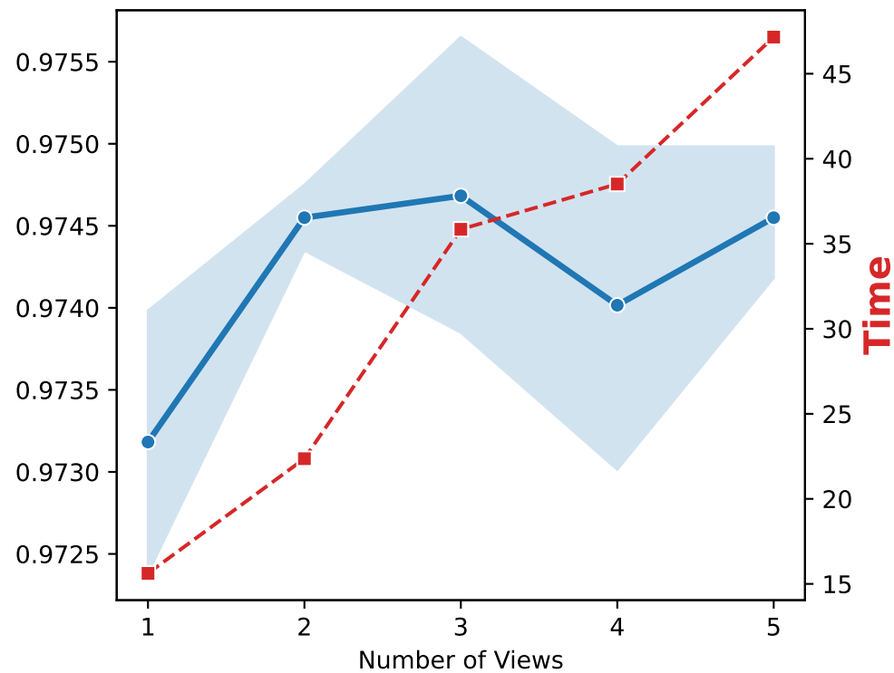
Dataset: VID
