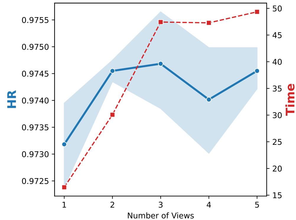
Dataset: VID
