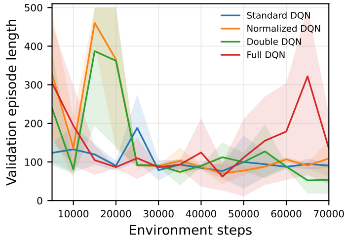
DQN variants
