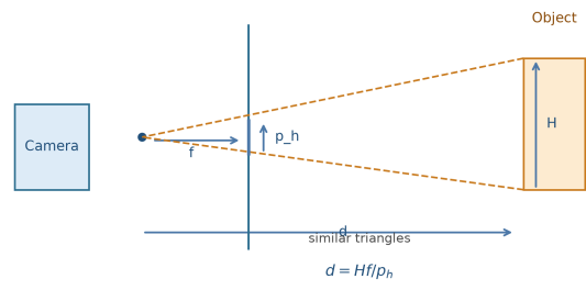
图 2: 单目距离估计的几何示意图
