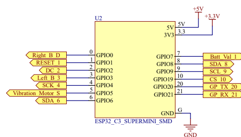
Microcontroller(ESP32 C3 Super-mini)
