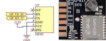
GPS Module
