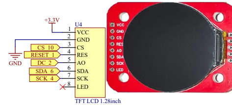
Display
