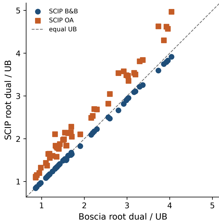
Optimized Boscia
