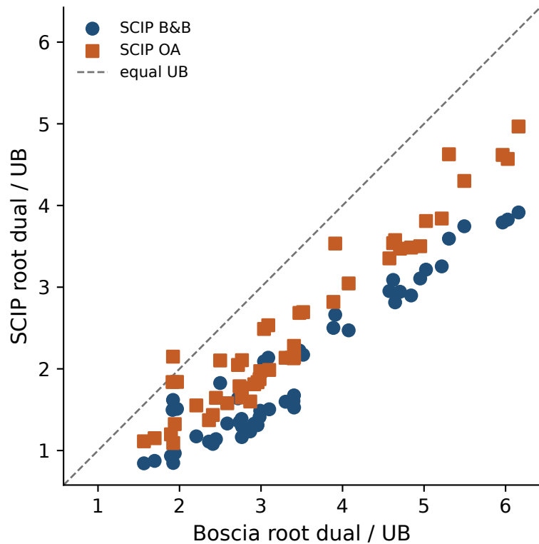
Baseline Boscia
