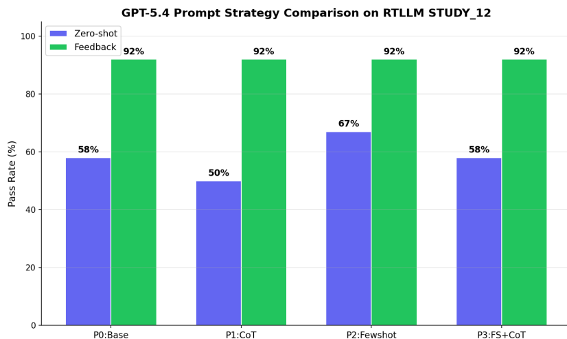
图 5.8 提示词策略零样本与反馈对比
