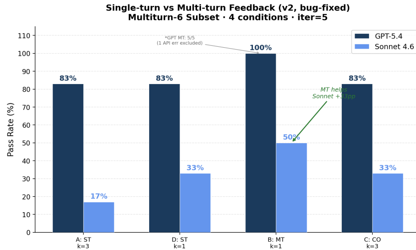
图 5.7 多轮对话反馈 v2 条件对比
