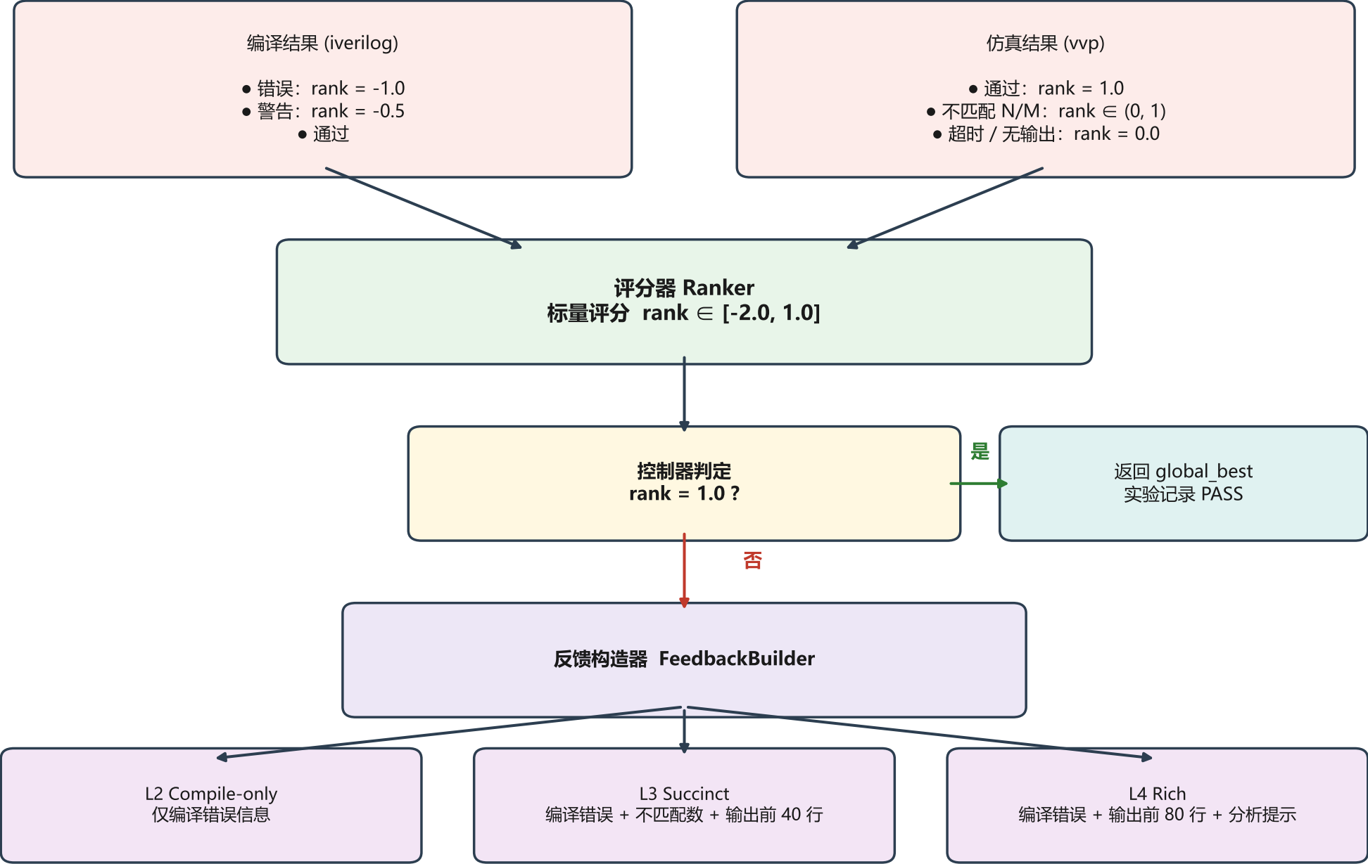
图 3.5 EDA 验证结果到反馈提示词的转换逻辑
