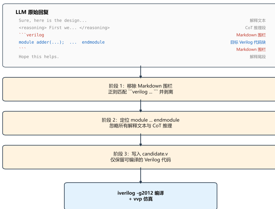
图 3.4 LLM 回复到可编译 Verilog 的提取流程
