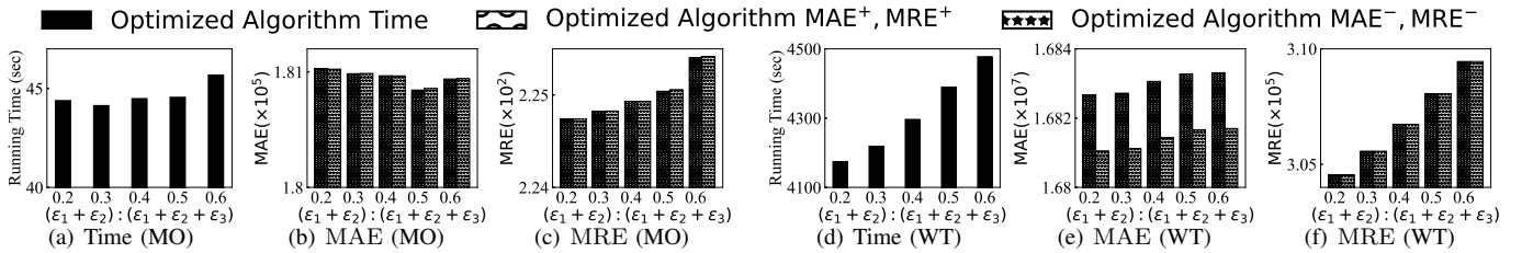
Fig. 14: Impact of privacy budget allocation (\epsilon_1 + \epsilon_2) : (\epsilon_1 + \epsilon_2 + \epsilon_3)
