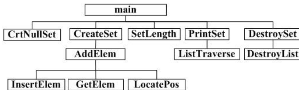
图 4-1 函数间的调用关系
