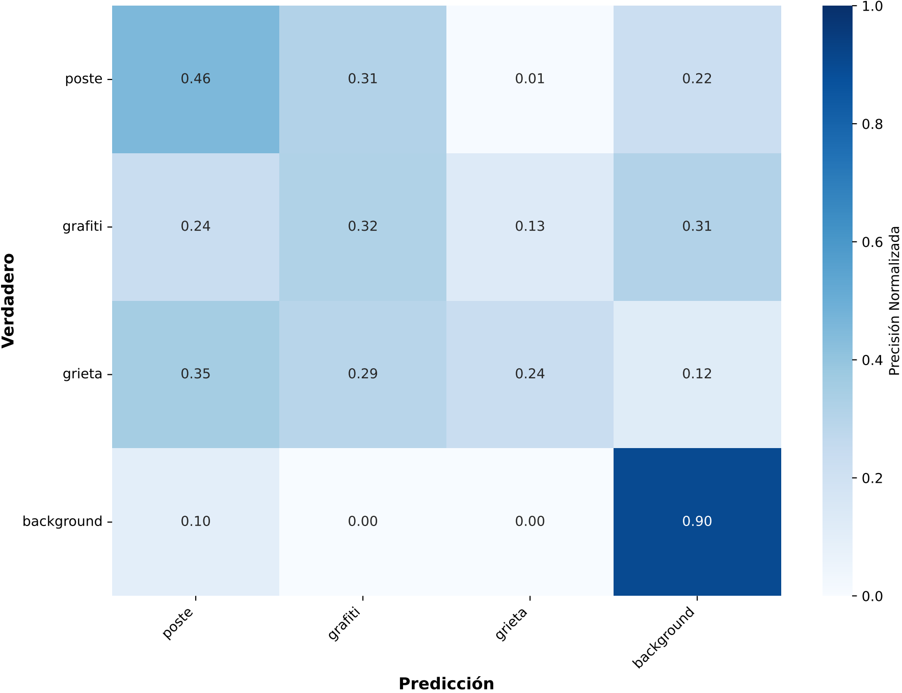
Matriz de Confusión Normalizada - Entrenamiento 1 (Versión Alternativa)
