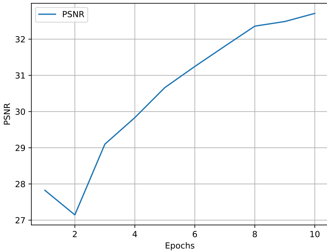
PSNR
