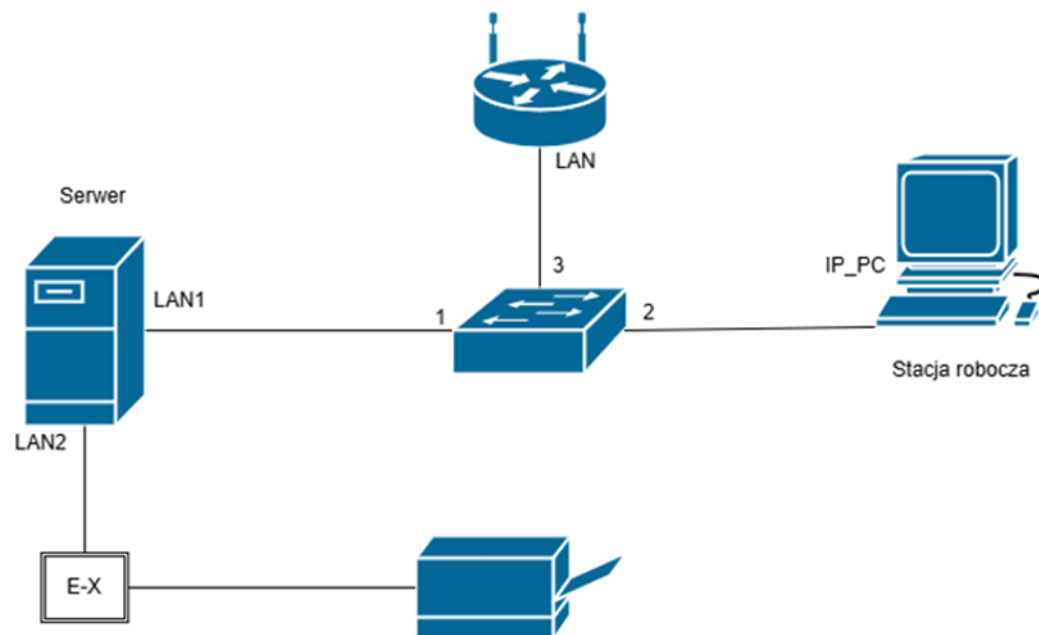
Załącznik 1. Schemat połączenia urządzeń
