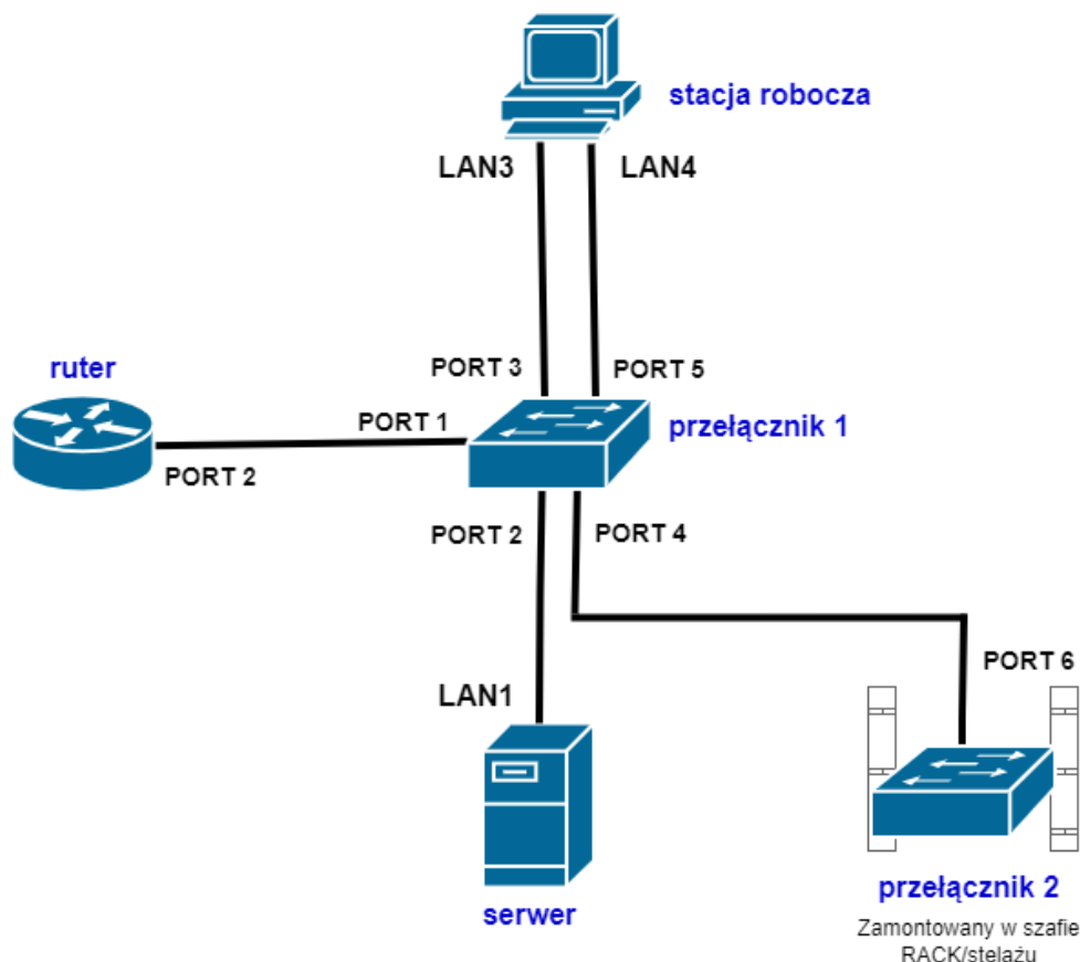
Schemat połączenia urządzeń
