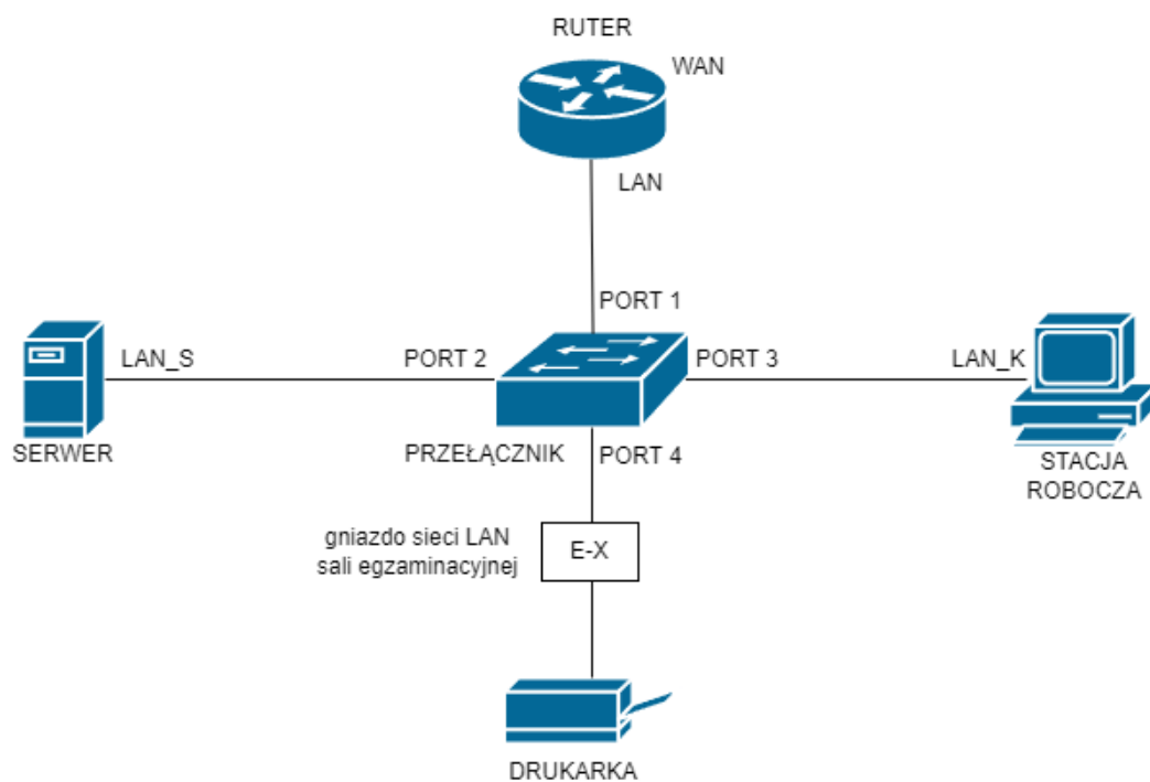
Schemat połączenia urządzeń
