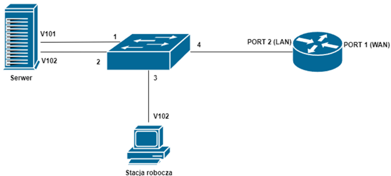
Załącznik 1. Schemat połączenia urządzeń
