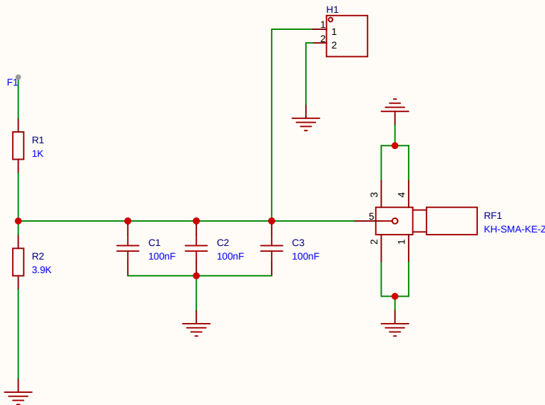
分压检测电路
