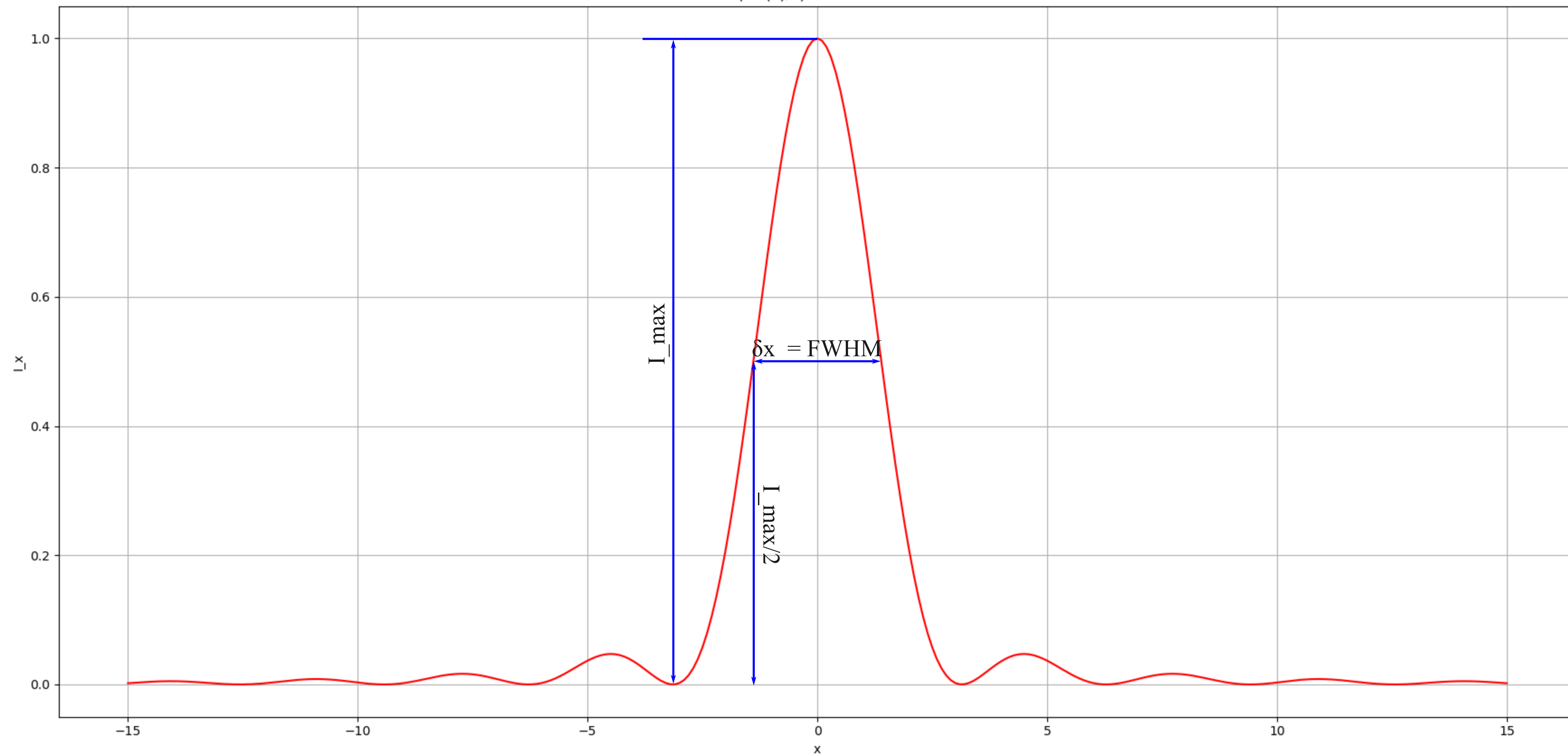
(\sin(x)/x)^2 function
