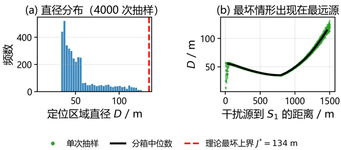
图 11 左：按本文规则选取第二检测点后，定位区域直径的 Monte-Carlo 分布（4000 次），红色虚线为最坏情形上界 J^* = 134 \text{ m} ，无一次越界；右：直径与真实源距离的关系，最大值出现在 r = 1500 \text{ m} 处，与理论分析一致
