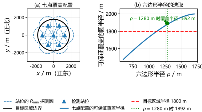
图 13 左：中心 + 正六边形顶点共 7 个检测位置（三角）的 R_{\min} = 1000 \text{ m} 探测圆（虚线）覆盖整个目标域（黑实线圆）；右：七点配置的覆盖半径随六边形半径 \rho 的变化， \rho = 1280 \text{ m} 时达到 1892 m ，满足 \geq 1800 \text{ m}
