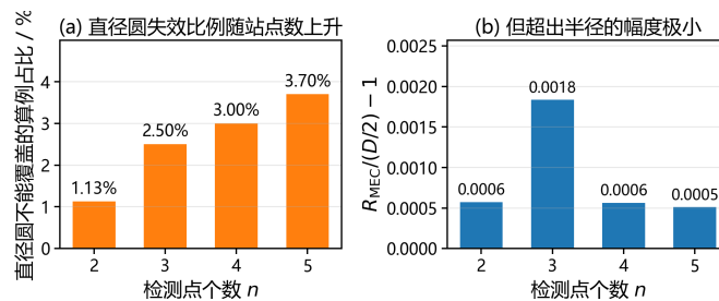
图 5 左: 直径圆不能覆盖定位区域的算例比例; 右: 超出半径的相对量级 (最大仅 0.18%)
