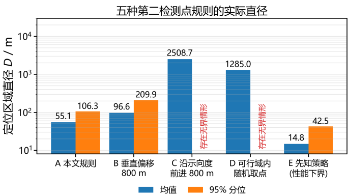
图 10 五种第二检测点规则的实际定位区域直径（纵轴取对数坐标；C、D 两策略在部分算例中定位区域无界，其 95% 分位为 \infty ，故仅给出均值）
