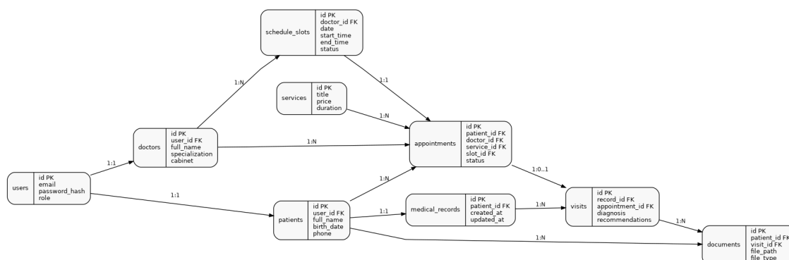
Рисунок 2.2 – Упрощённая ER-диаграмма базы данных
