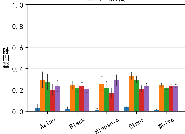
LR / 族裔
