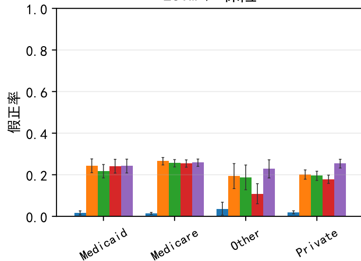
LSTM / 保险
