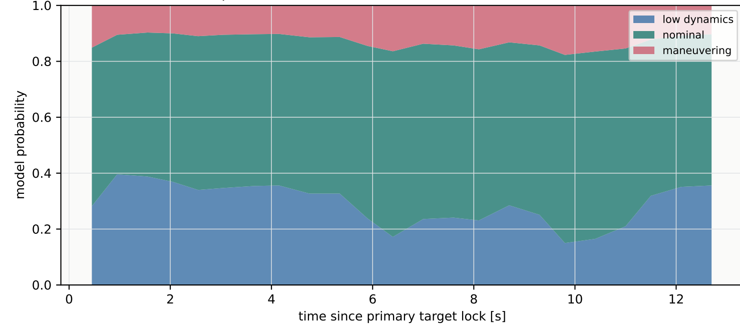
(d) Three-model IMM posterior
