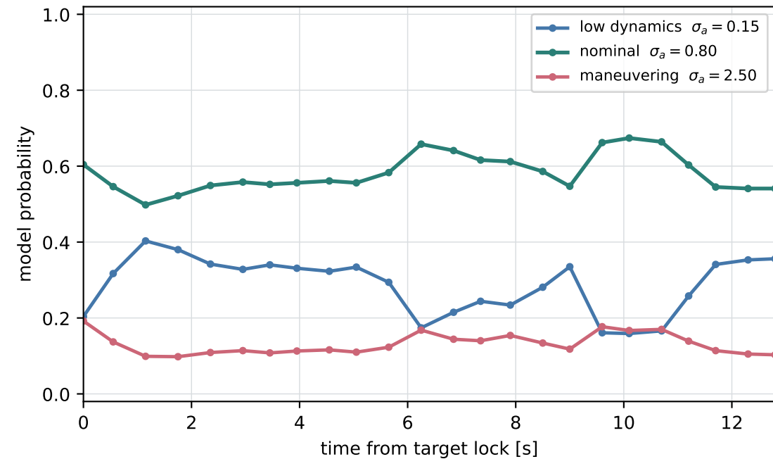
(d) Three-model IMM probability evolution
