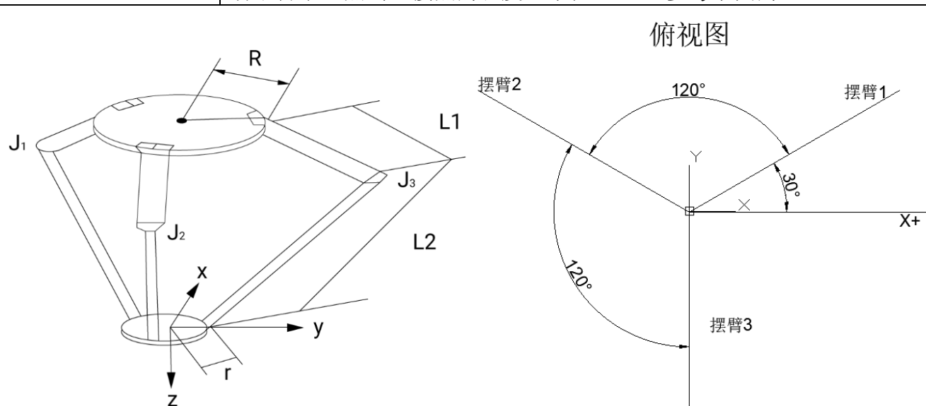
Delta 机械臂结构图
