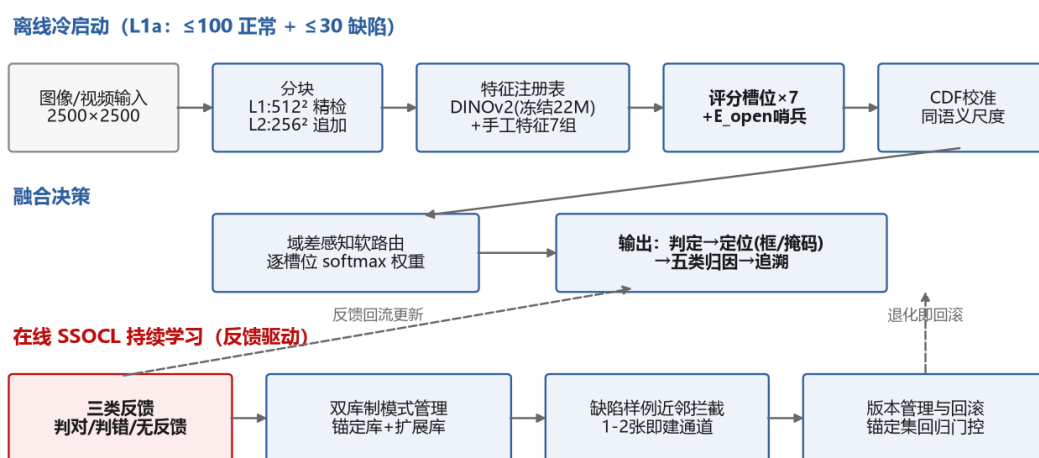
可自学习 AOI 实时在线 AI 质检系统 · 总体架构
