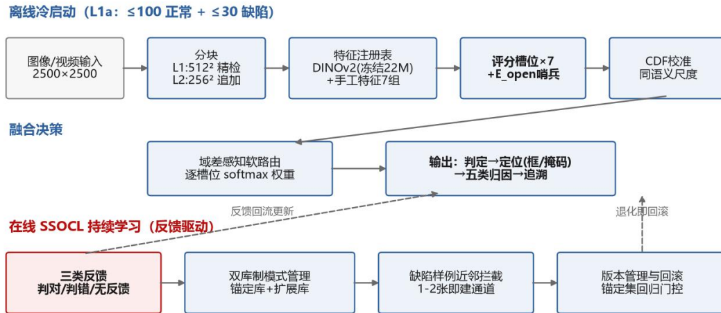
可自学习 AOI 实时在线 AI 质检系统·总体架构
