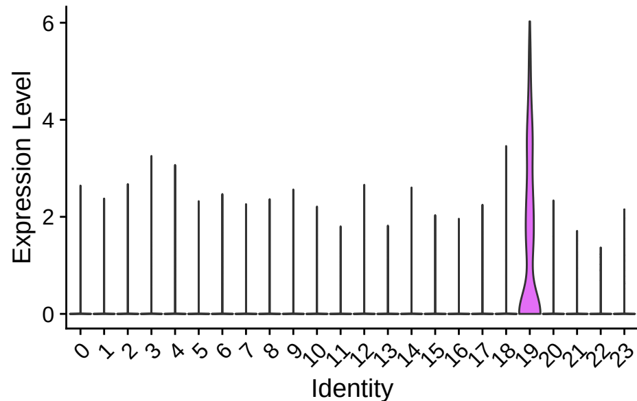
XLOC-001150#SVEP1-RAT#P0C6B8
