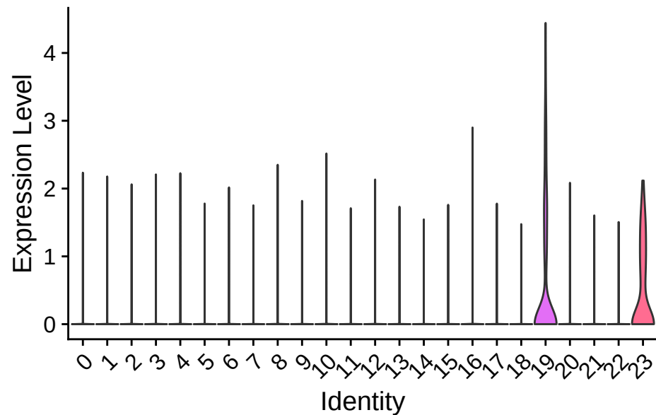
XLOC-001150#SVEP1-RAT#P0C6B8
