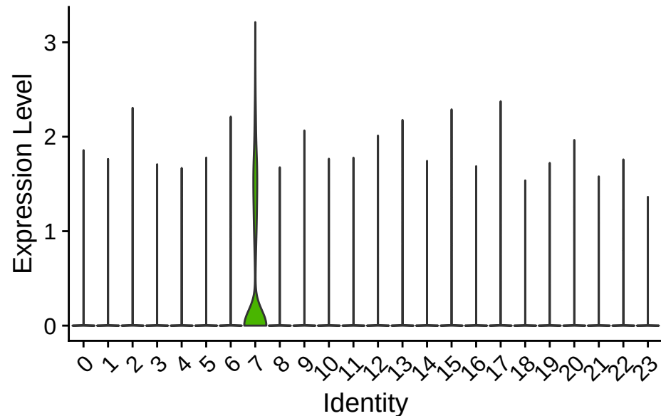
gene-evm.model.ptg000001l.686#SOX14-DANRE#Q32PP9
