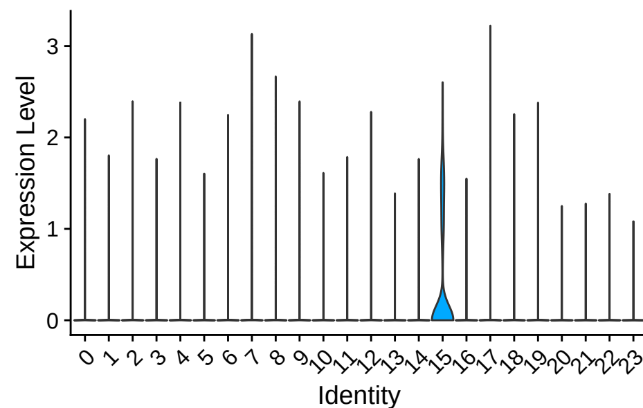
gene-evm.model.ptg000022l.585#ACH1-CAEEL#P48180
