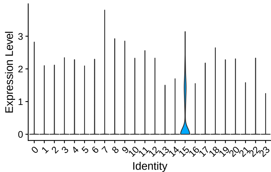
gene-evm.model.ptg000001l.686#SOX14-DANRE#Q32PP9
