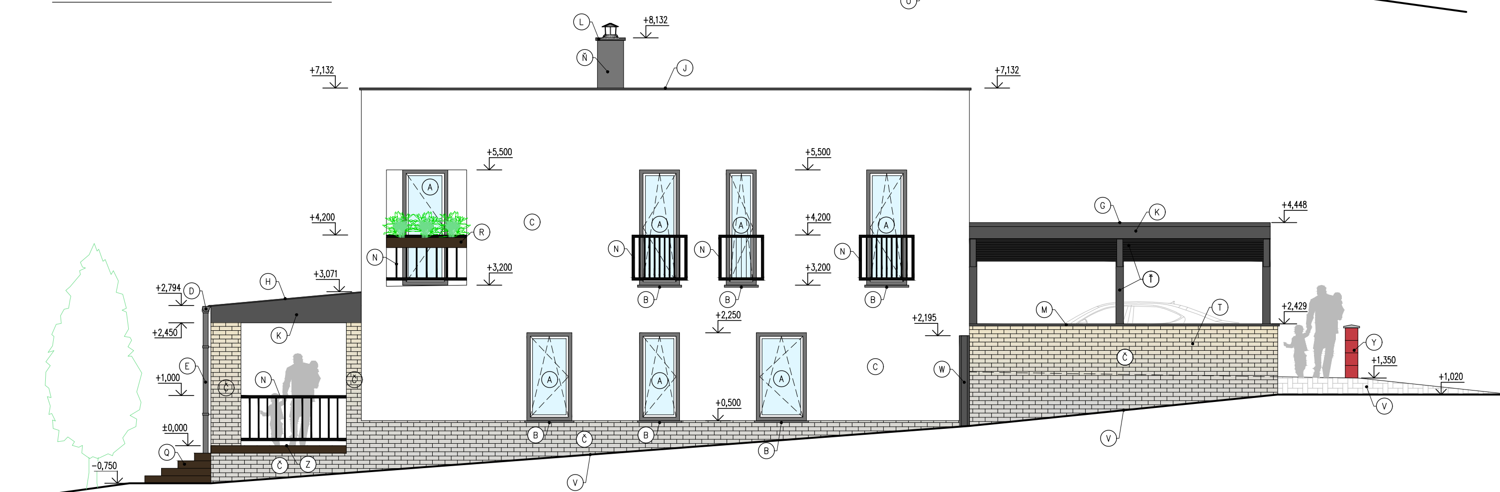
SEVEROZÁPADNÝ POHĽAD
