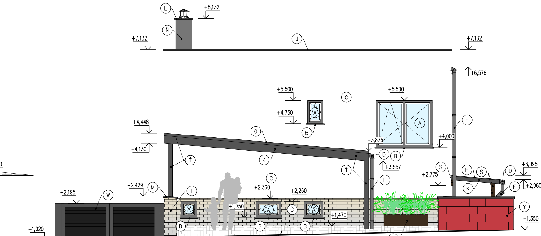
SEVEROVÝCHODNÝ POHĽAD
