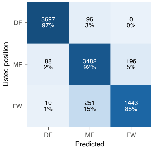
Multinomial logistic acc 0.931, macro F1 0.918
