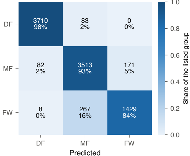
LightGBM acc 0.934, macro F1 0.921
