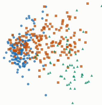
PCA
