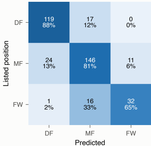
Multinomial logistic acc 0.811, macro F1 0.786
