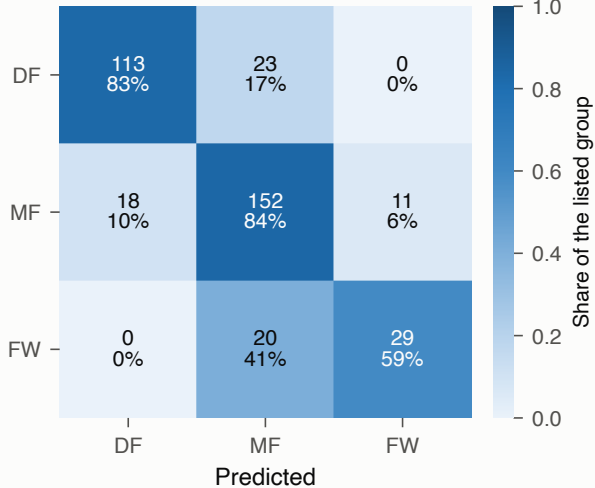
LightGBM acc 0.803, macro F1 0.769
