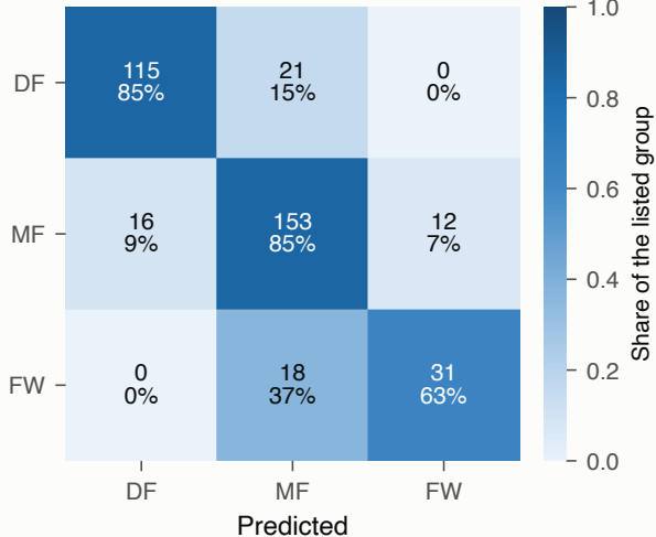
LightGBM acc 0.817, macro F1 0.785
