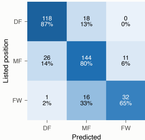
Multinomial logistic acc 0.803, macro F1 0.779
