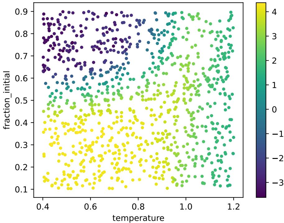
corr2d: log10 eta used (Laplacian)
