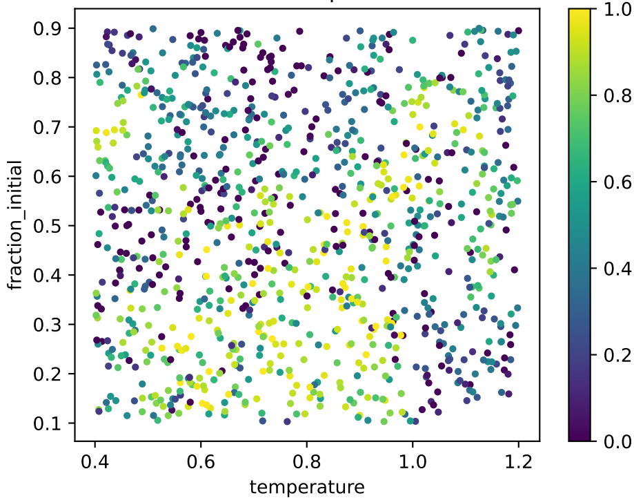
corr2d: local LLE explained fraction
