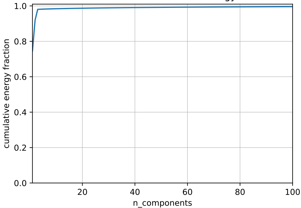
Global PCA cumulative energy
