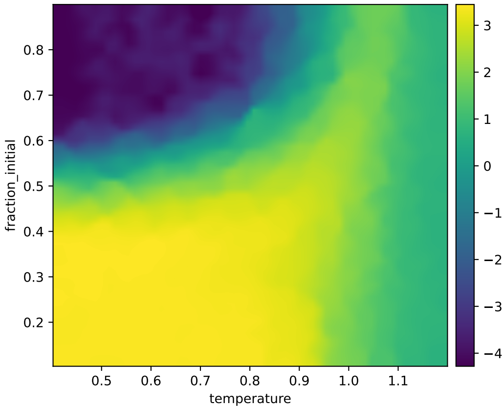
corr2d: heatmap log10 eta used
