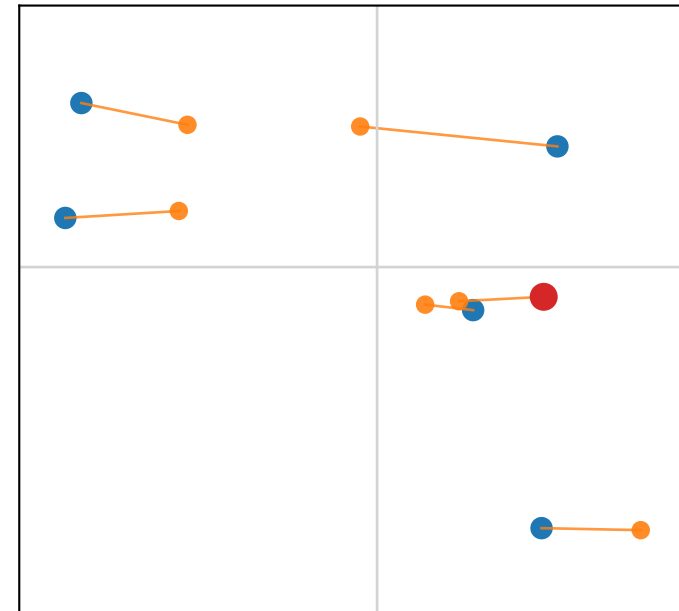
B) 3) LOO residuals (e=0.00)
