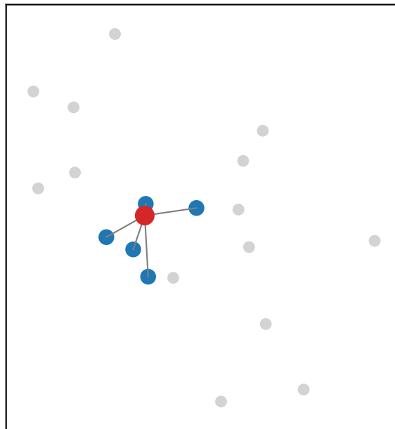
B) 2) kNN in Y
