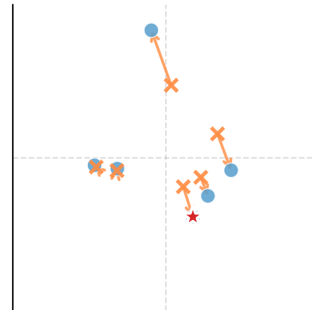
(4) LOO Score: 0.000
