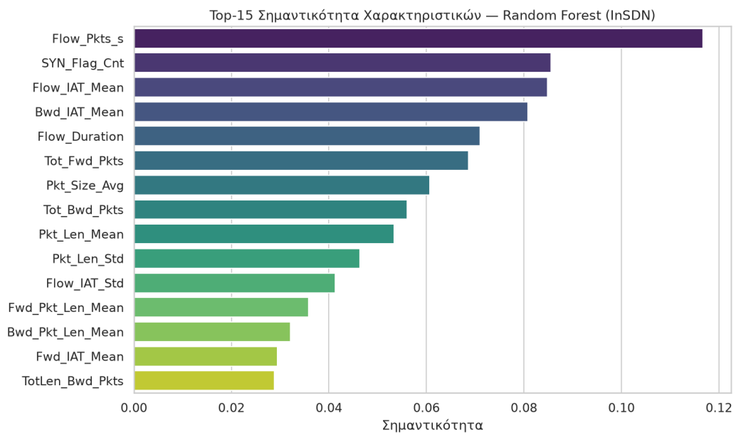
Σχήμα 6-30: Σημαντικότητα χαρακτηριστικών (thesis έκδοση).
