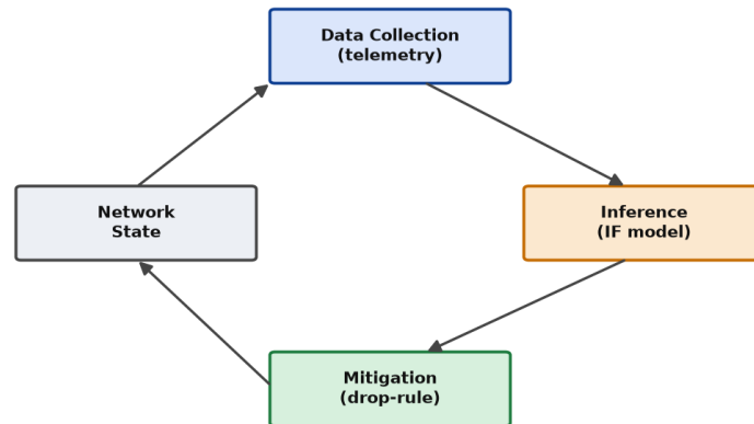
Σχήμα 5-3: Ο κλειστός βρόχος εποπτείας-απόφασης-δράσης.
