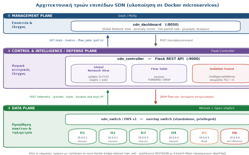
Σχήμα 5-1: Σχηματική αναπαράσταση της αρχιτεκτονικής του συστήματος.
