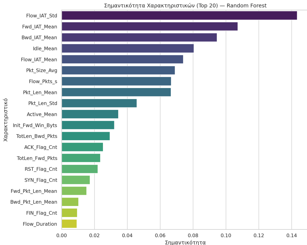
Σχήμα 7: Σημαντικότητα των σημαντικότερων χαρακτηριστικών κατά το Random Forest.
