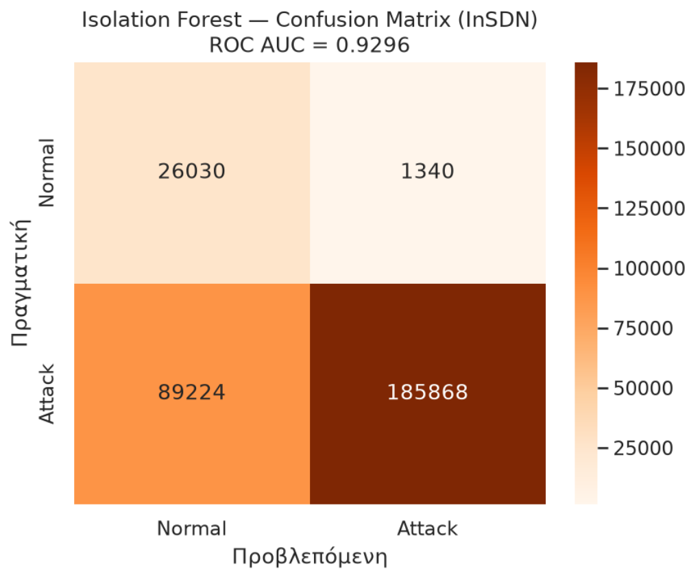
Σχήμα 18: Πίνακας σύγκρισης του Isolation Forest.
