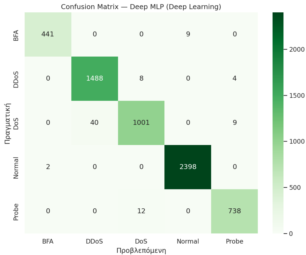
Σχήμα 14: Πίνακας σύγχυσης του μοντέλου Deep MLP.
