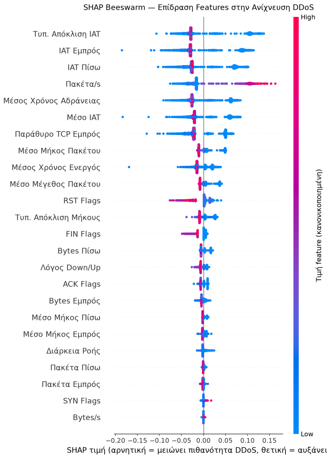
Σχήμα 8: Διάγραμμα SHAP (beeswarm), κατεύθυνση και μέγεθος επίδρασης ανά χαρακτηριστικό.
