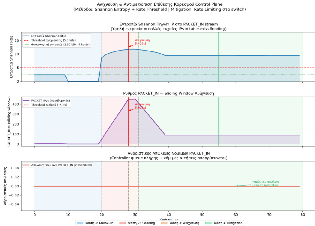
Σχήμα 25: Ανίχνευση της επίθεσης κορεσμού μέσω εντροπίας Shannon.
