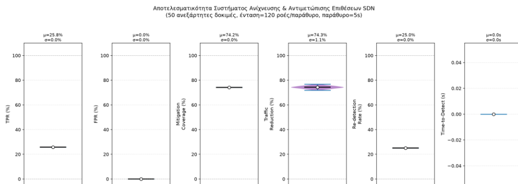
Σχήμα 22: Κατανομές (violin plots) των μετρικών αποτελεσματικότητας αντιμετώπισης.
