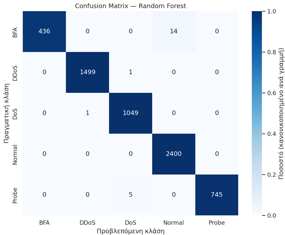
Σχήμα 6: Πίνακας σύγχυσης του βέλτιστου κλασικού μοντέλου (Random Forest).
