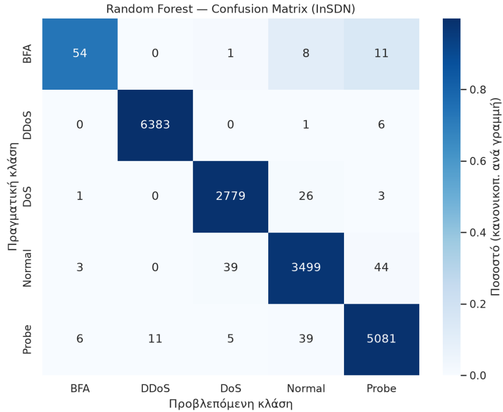
Σχήμα 33: Πίνακας σύγχυσης του Random Forest (thesis έκδοση).
