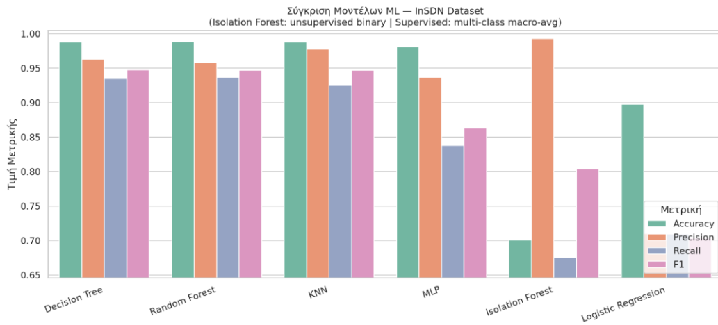
Σχήμα 35: Συγκριτική απόδοση μοντέλων (thesis έκδοση).
