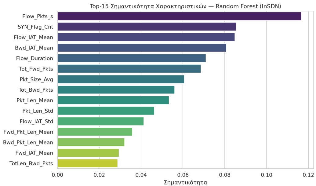
Σχήμα 34: Σημαντικότητα χαρακτηριστικών (thesis έκδοση).
