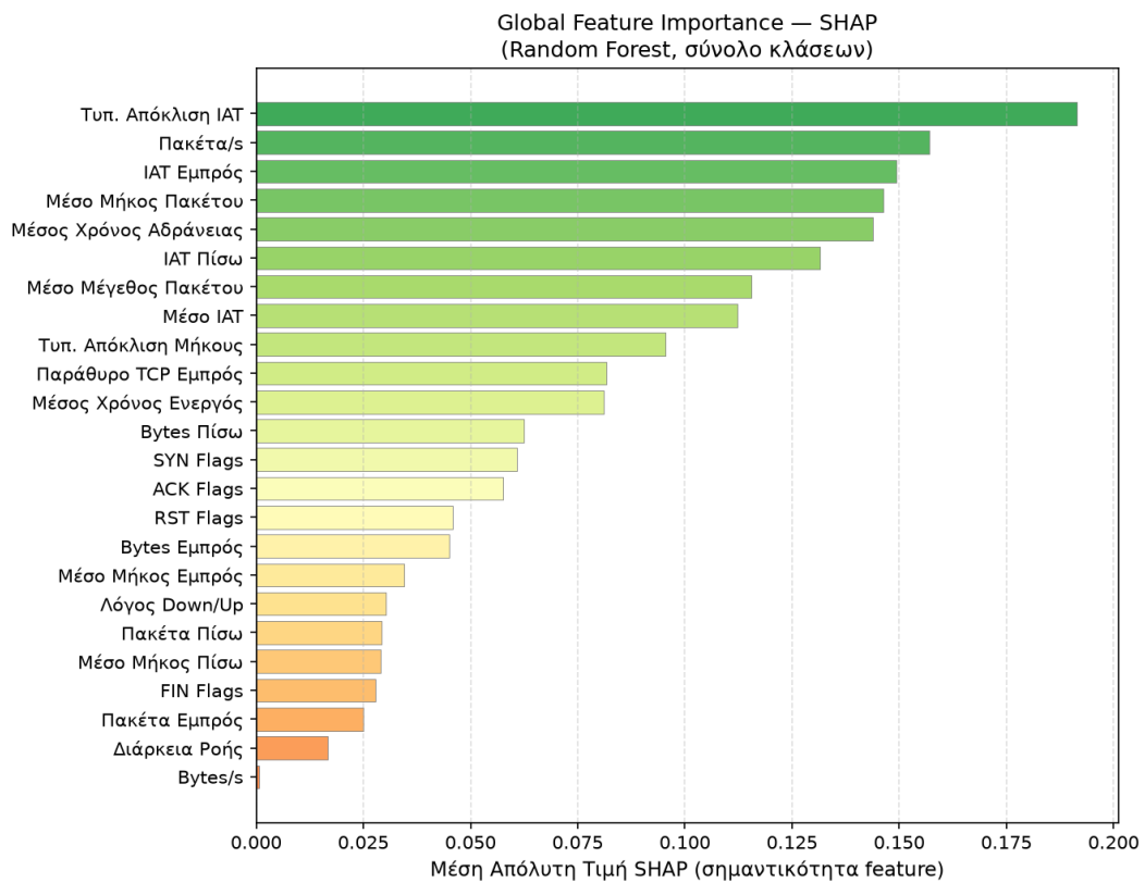
Σχήμα 9: Global σημαντικότητα χαρακτηριστικών κατά SHAP (μέση απόλυτη τιμή).
