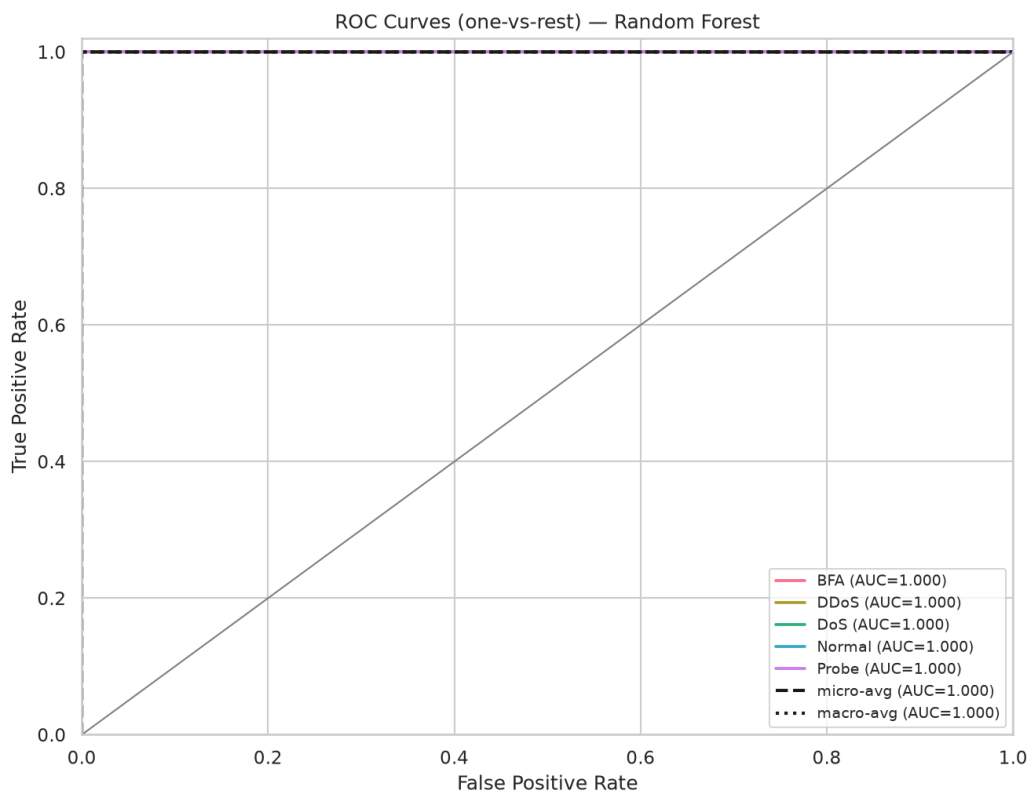
Σχήμα 11: Καμπύλες ROC ανά κατηγορία επίθεσης (one-vs-rest).
