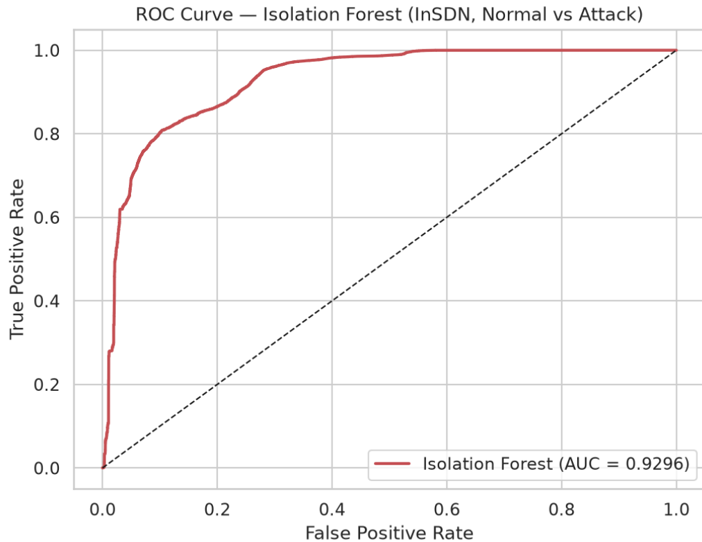
Σχήμα 19: Καμπύλη ROC του Isolation Forest.
