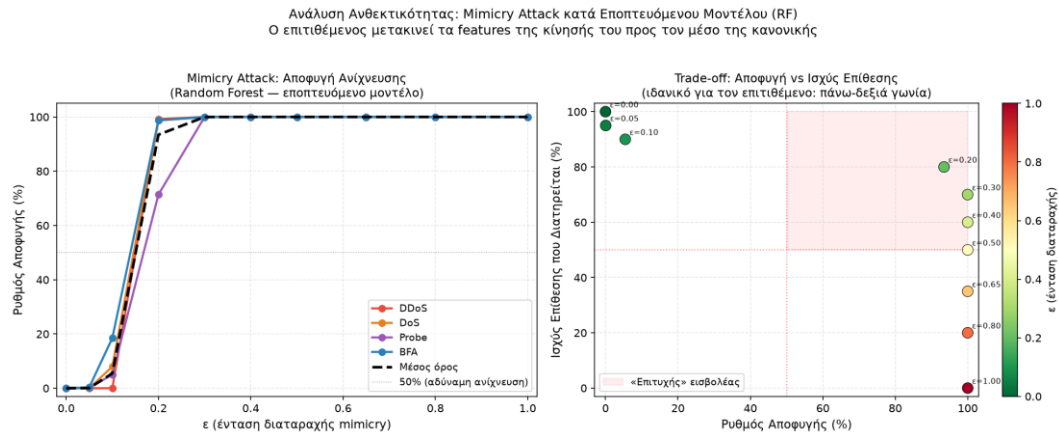
Σχήμα 28: Ρυθμός αποφυγής συναρτήσει της διαταραχής \epsilon (mimicry εναντίον Random Forest) και το trade-off ισχύος επίθεσης.
