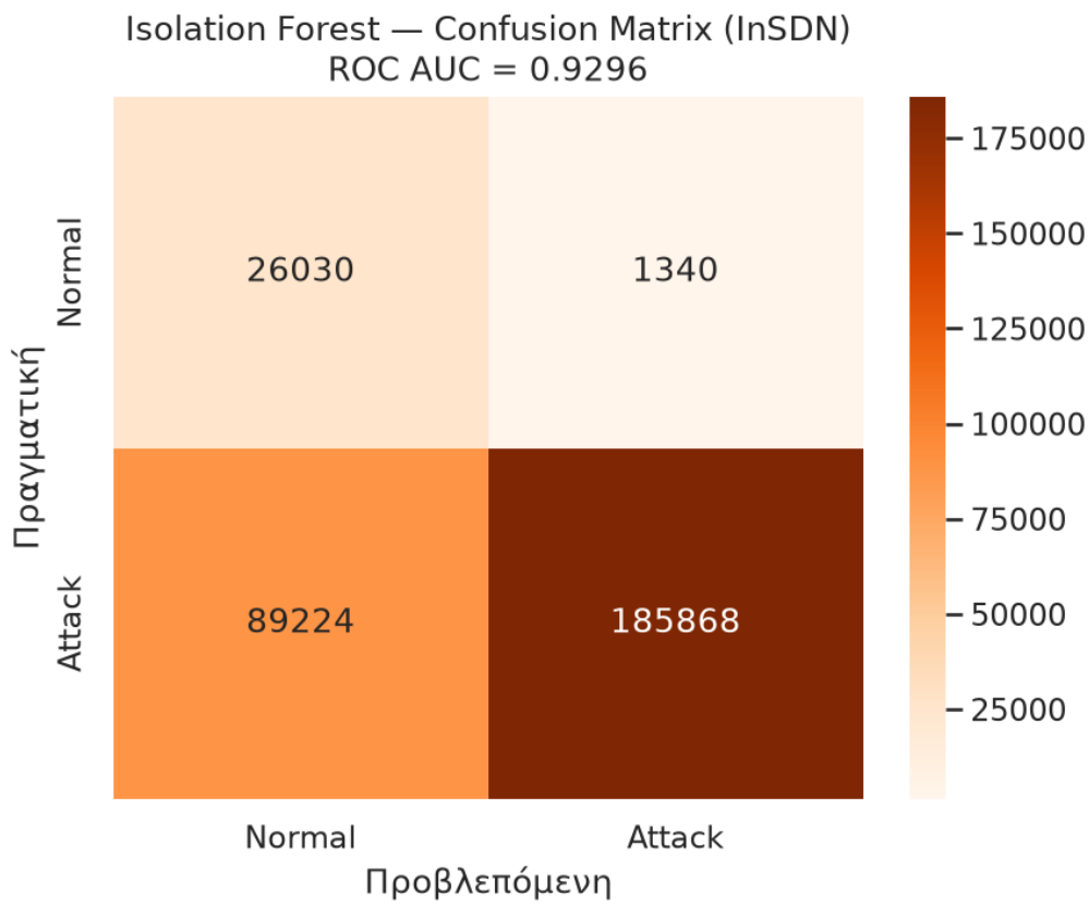
Σχήμα 18: Πίνακας σύγχυσης του Isolation Forest.
