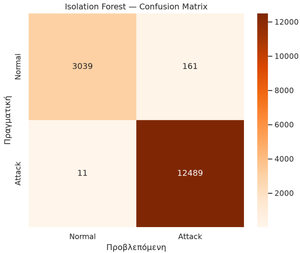
Σχήμα 31: Εναλλακτικός πίνακας σύγκρισης του Isolation Forest .
