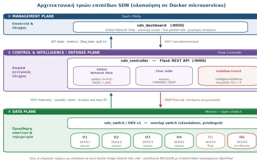
Σχήμα 1: Σχηματική αναπαράσταση της αρχιτεκτονικής του συστήματος.
