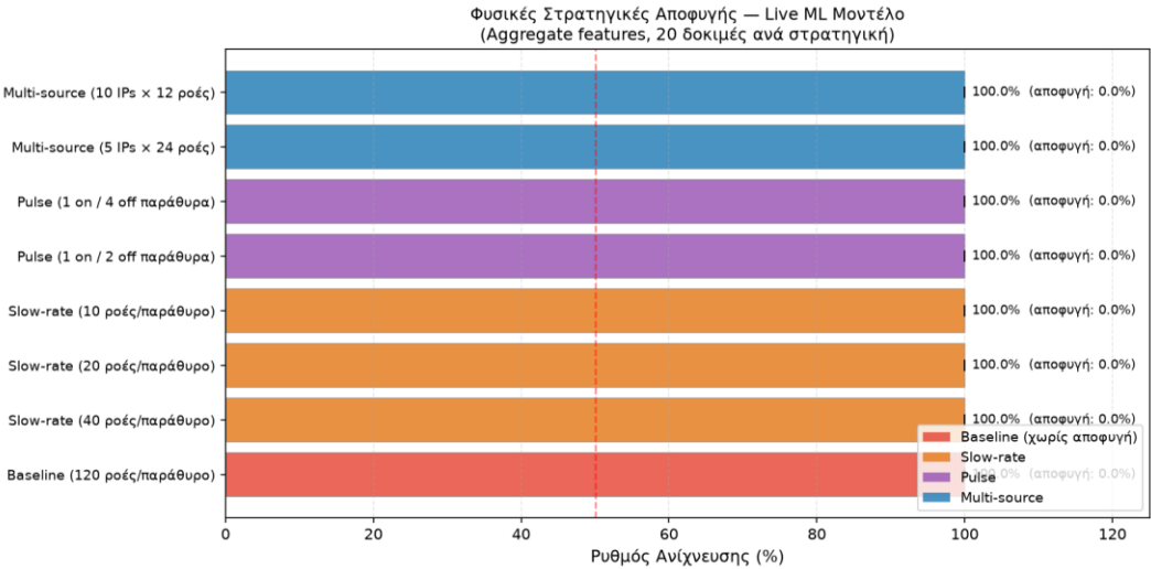
Σχήμα 30: Φυσικές στρατηγικές αποφυγής εναντίον του ζωντανού μοντέλου.
