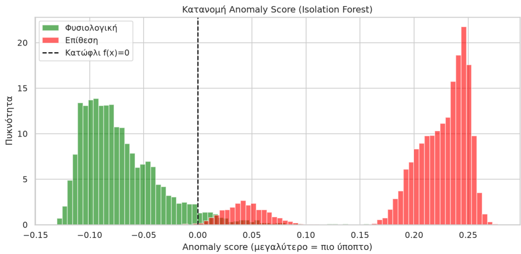
Σχήμα 32: Κατανομή anomaly scores του Isolation Forest .
