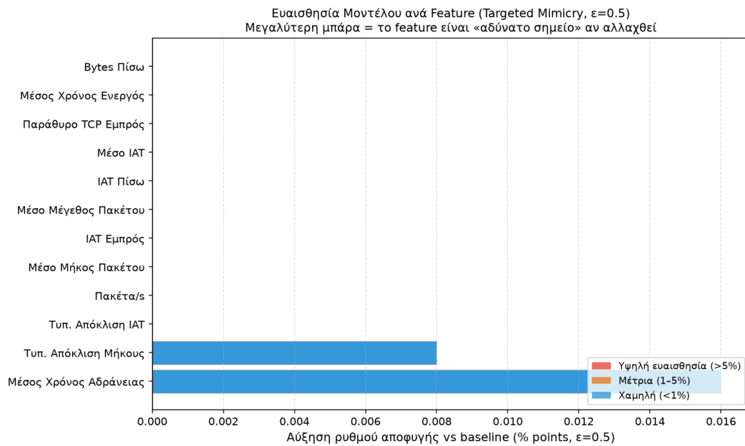
Σχήμα 29: Ευαισθησία ανά χαρακτηριστικό (στοχευμένη μίμηση).
