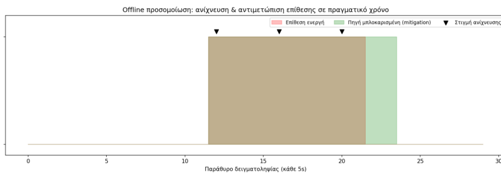
Σχήμα 36: Χρονολόγιο offline replay: ανίχνευση επίθεσης σε επανάληψη καταγεγραμμένης κίνησης.
