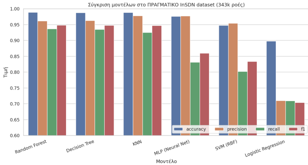
Σχήμα 16: Σύγκριση μοντέλων στο πραγματικό σύνολο δεδομένων InSDN.
