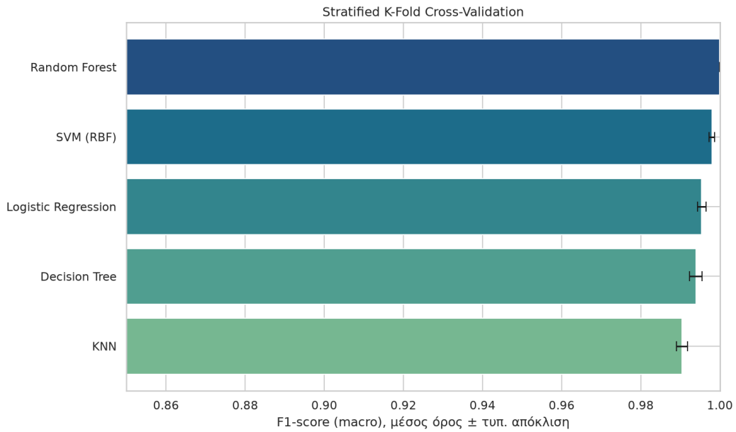
Σχήμα 12: Διασταυρούμενη επικύρωση 5-fold: F1 -score (μέσος \pm τυπική απόκλιση).
