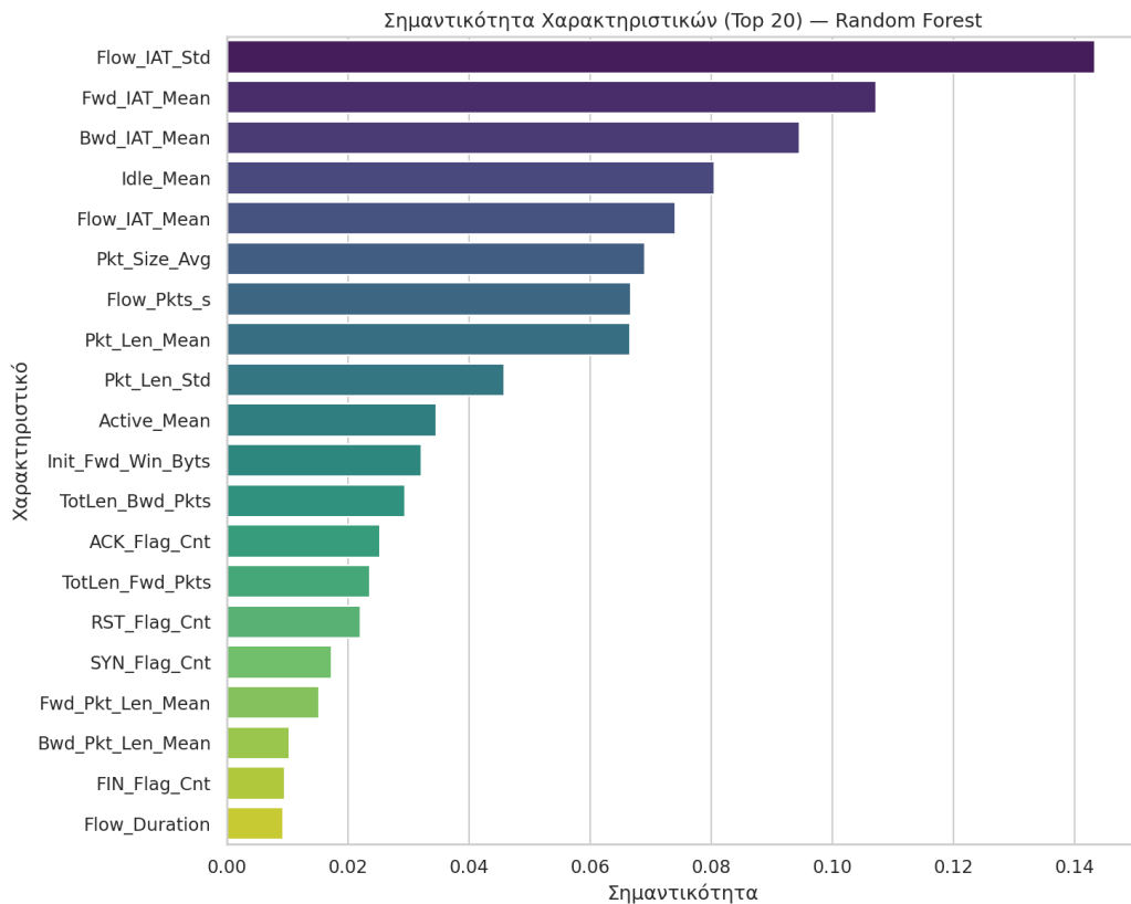
Σχήμα 7: Σημαντικότητα των σημαντικότερων χαρακτηριστικών κατά το Random Forest.
