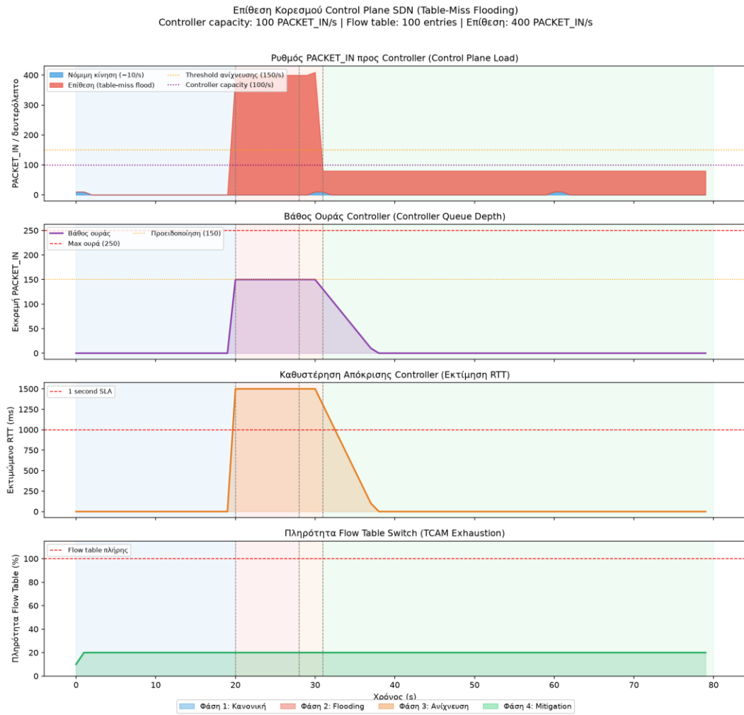
Σχήμα 24: Επισκόπηση της επίθεσης κορεσμού control plane (ρυθμός Packet-In, ουρά, RTT, πίνακας ροών).
