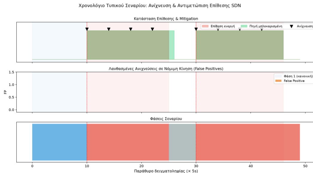
Σχήμα 23: Χρονολόγιο τυπικού σεναρίου αντιμετώπισης (ανίχνευση, αποκλεισμός, επανα-ανίχνευση).
