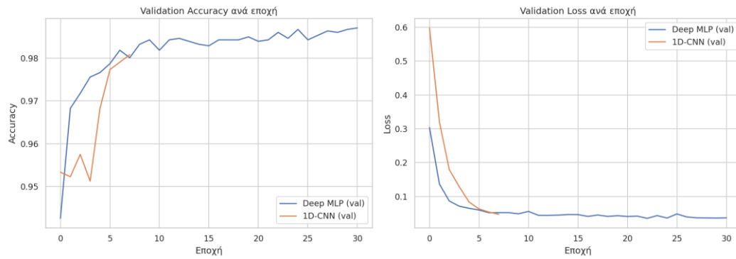
Σχήμα 15: Ιστορικό εκπαίδευσης των μοντέλων Βαθιάς Μάθησης (loss/accuracy ανά εποχή).
