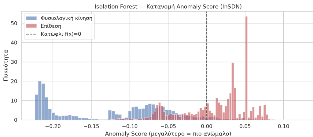
Σχήμα 20: Κατανομή anomaly scores του Isolation Forest για νόμιμη και κακόβουλη κίνηση.
