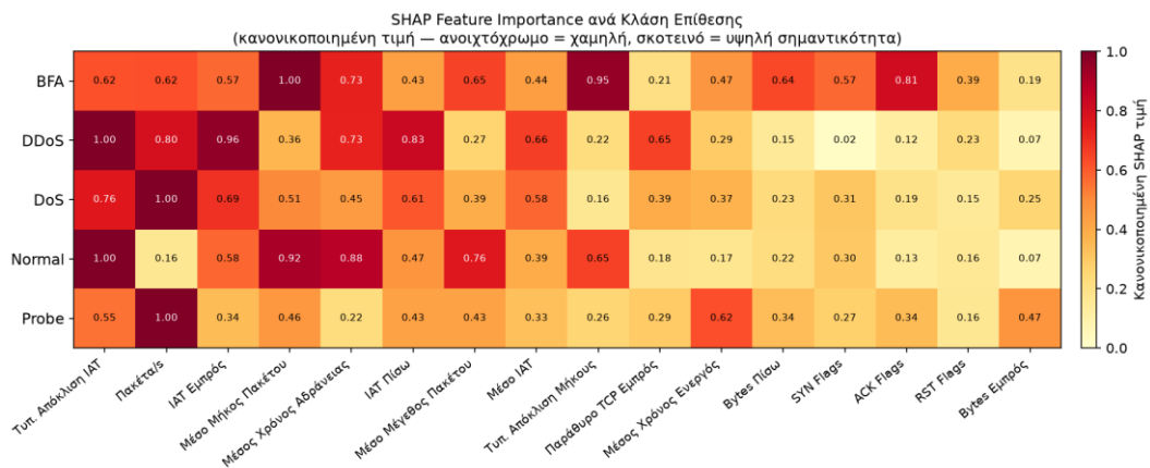
Σχήμα 10: Θερμικός χάρτης SHAP: ποια χαρακτηριστικά ανιχνεύουν ποια κατηγορία επίθεσης.
