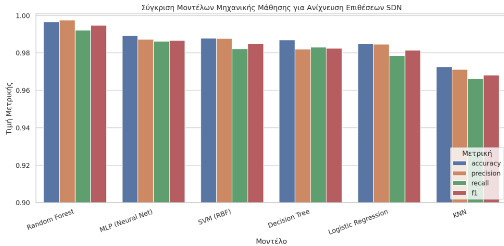
Σχήμα 5: Σύγκριση κλασικών μοντέλων Μηχανικής Μάθησης ως προς τις τέσσερις βασικές μετρικές.
