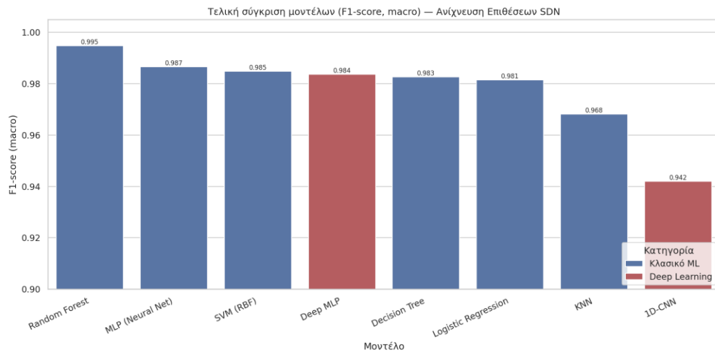
Σχήμα 13: Συνολική σύγκριση και των οκτώ μοντέλων (κλασικά και βαθιάς μάθησης).
