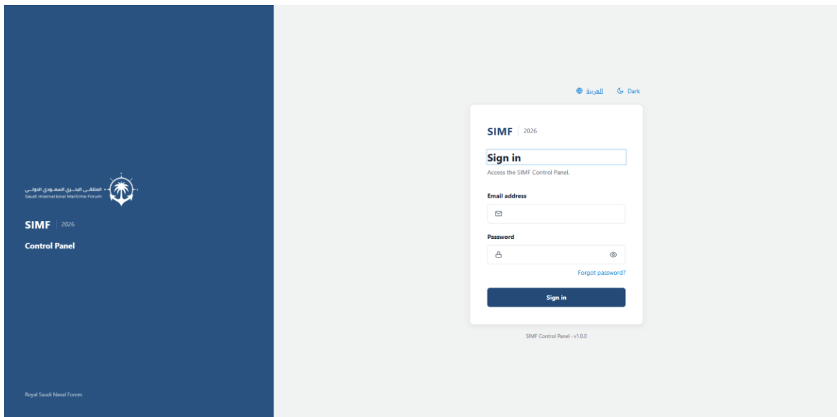
Figure 135 — /login
