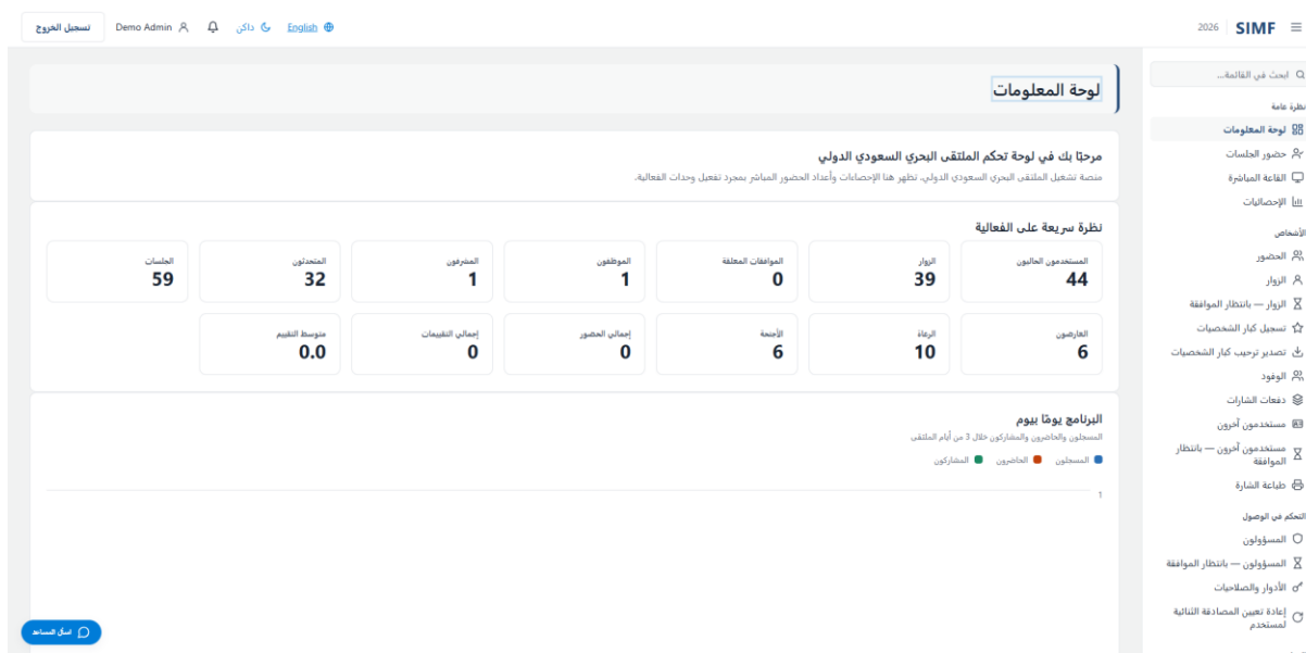
شكل 39 — لوحة المعلومات — /
