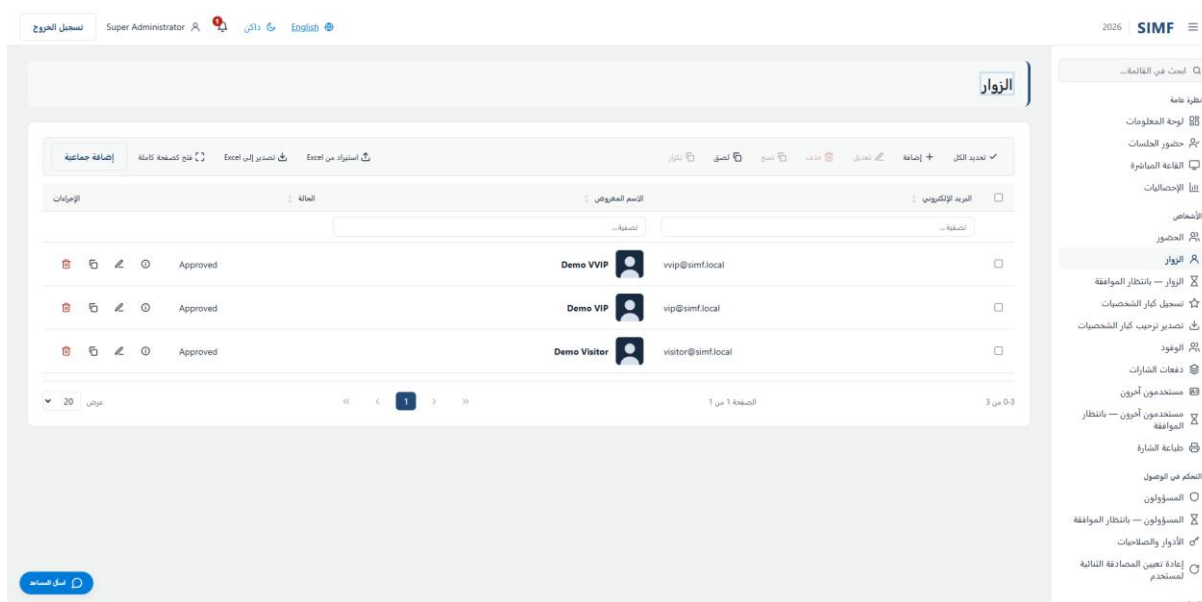
شكل 44 — الزوار — /admin/visitors
