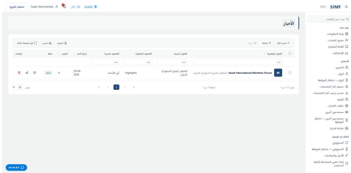
شكل 96 — الأخبار — /admin/news
