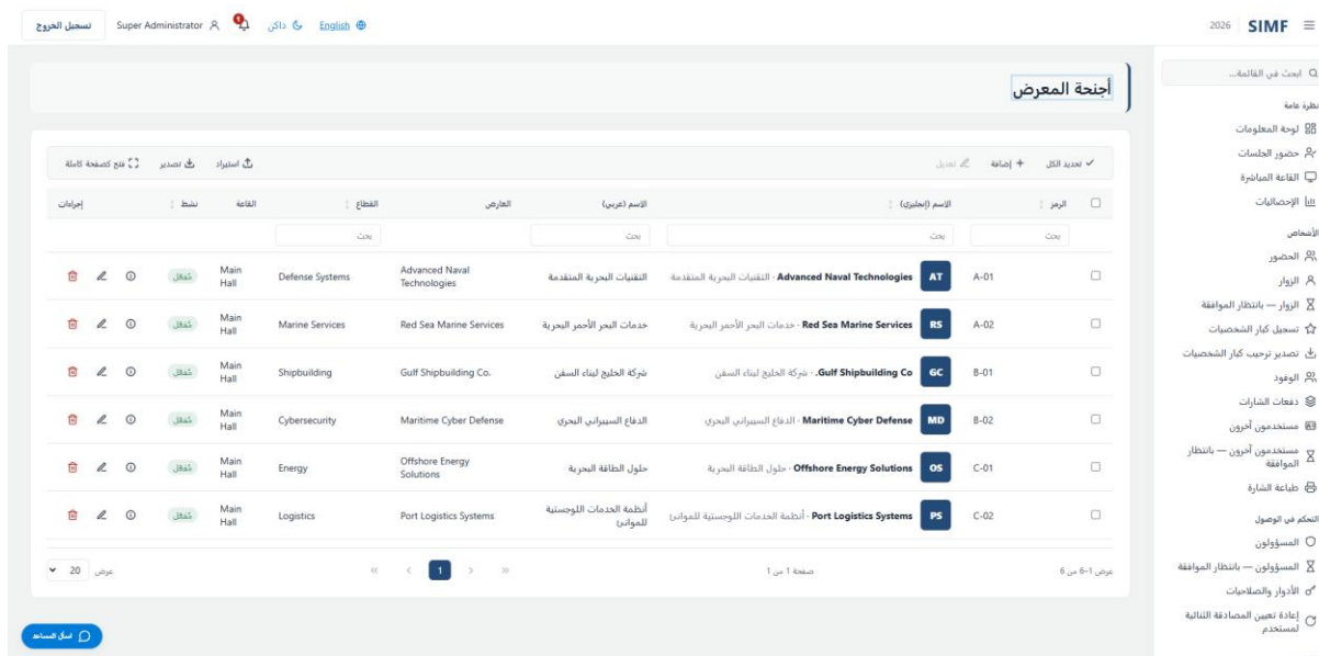
شكل 81 — الأجنحة — /admin/booths
