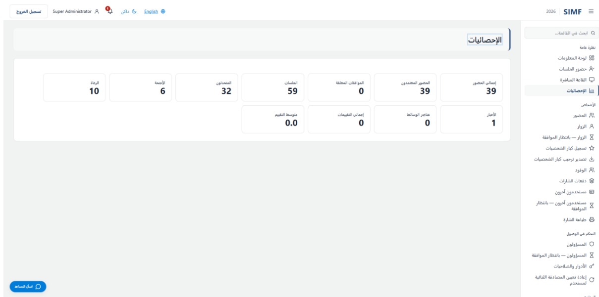
شكل 42 — الإحصائيات — /admin/statistics
