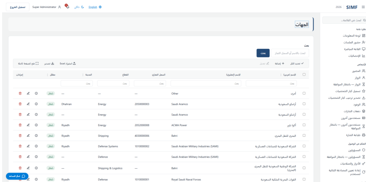
شكل 109 — الجهات — /admin/organisations
