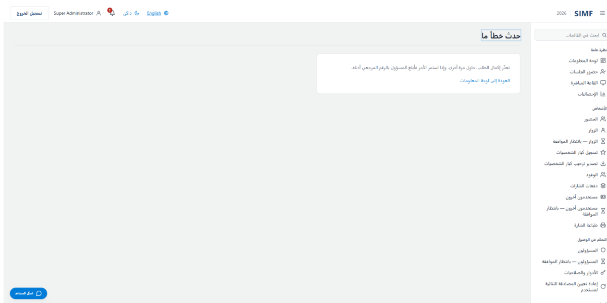
شكل 132 — /Error
