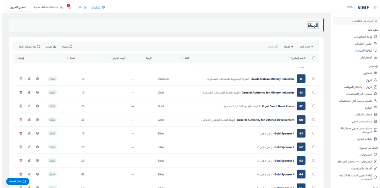
شكل 82 — الرعاة — /admin/sponsors
