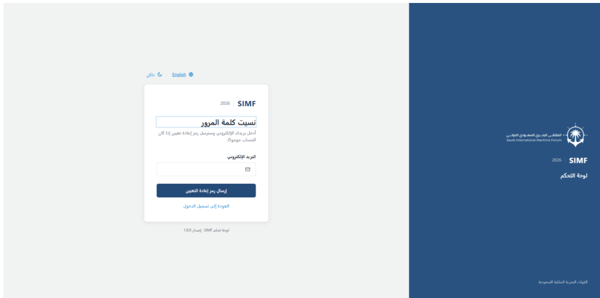
شكل 141 — /forgot-password
