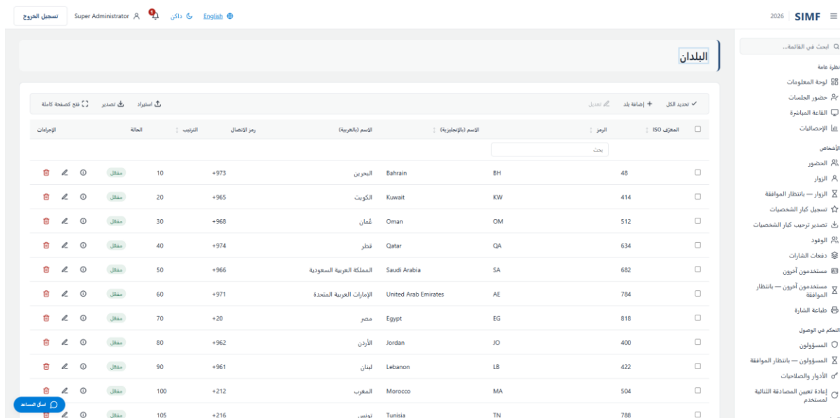
شكل 108 — البلدان — /admin/countries
