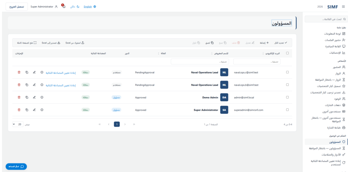
شكل 53 — المسؤولون — /admin/admins
