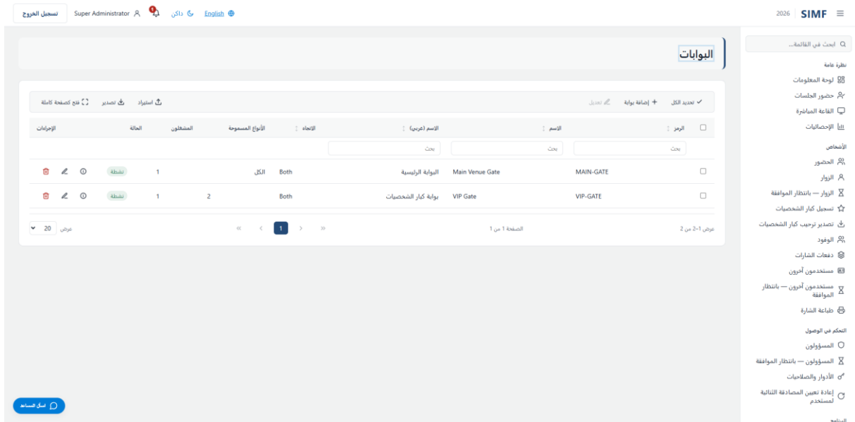
شكل 103 — البوابات — /admin/gates
