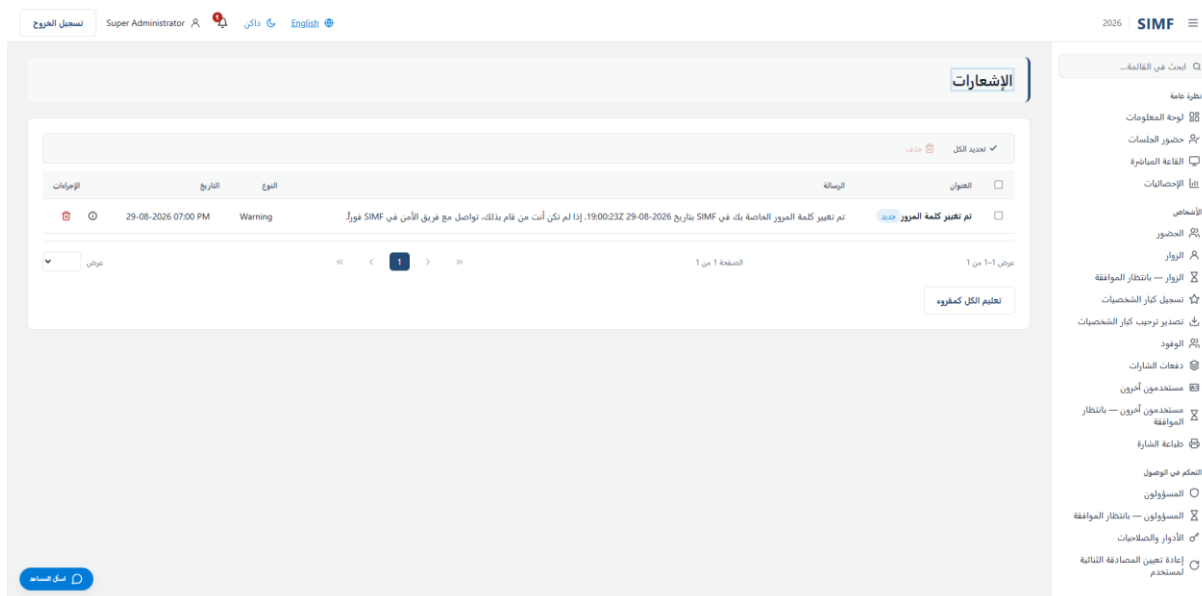
شكل 133 — /account/notifications
