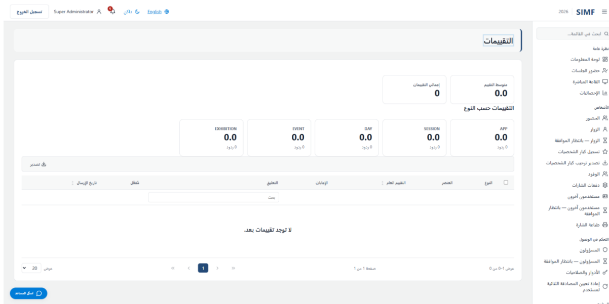
شكل 85 — التقييمات — /admin/ratings
