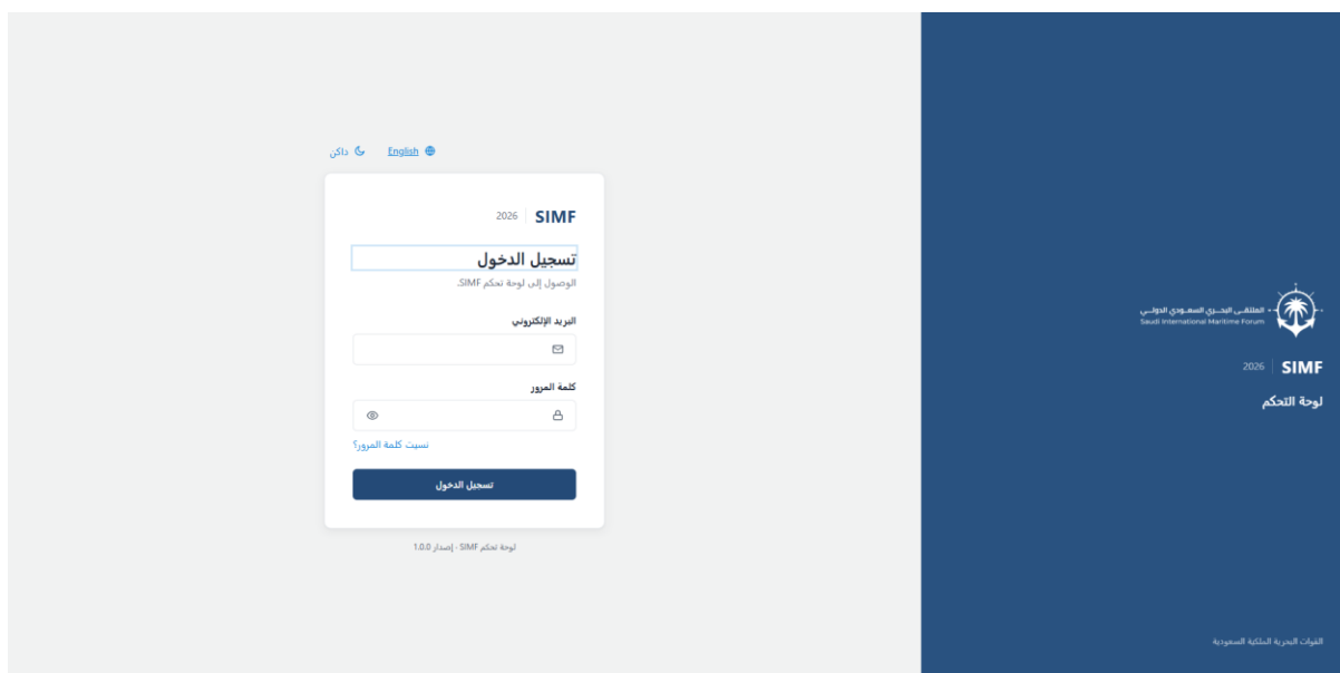
شكل 142 — /login
