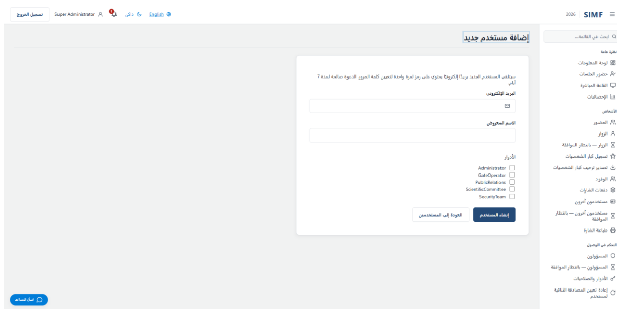
شكل 136 — /admin/admins/new
