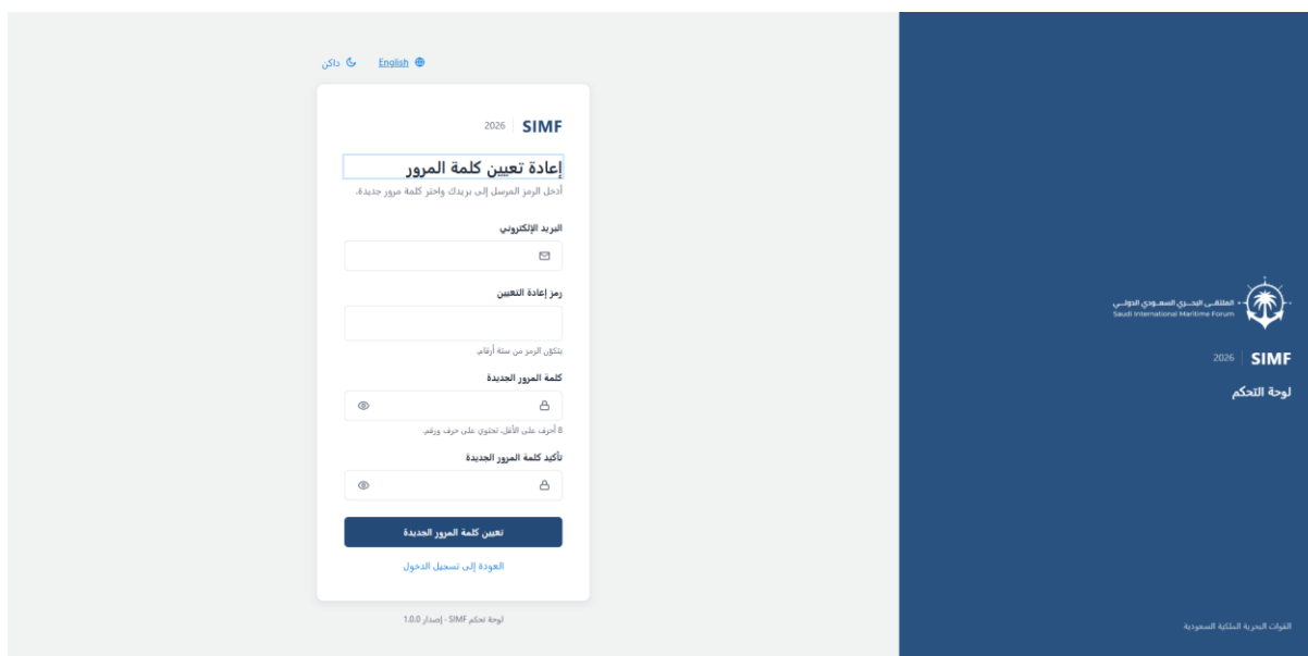
شكل 146 — /reset-password
