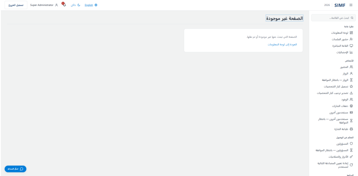
شكل 144 — /not-found
