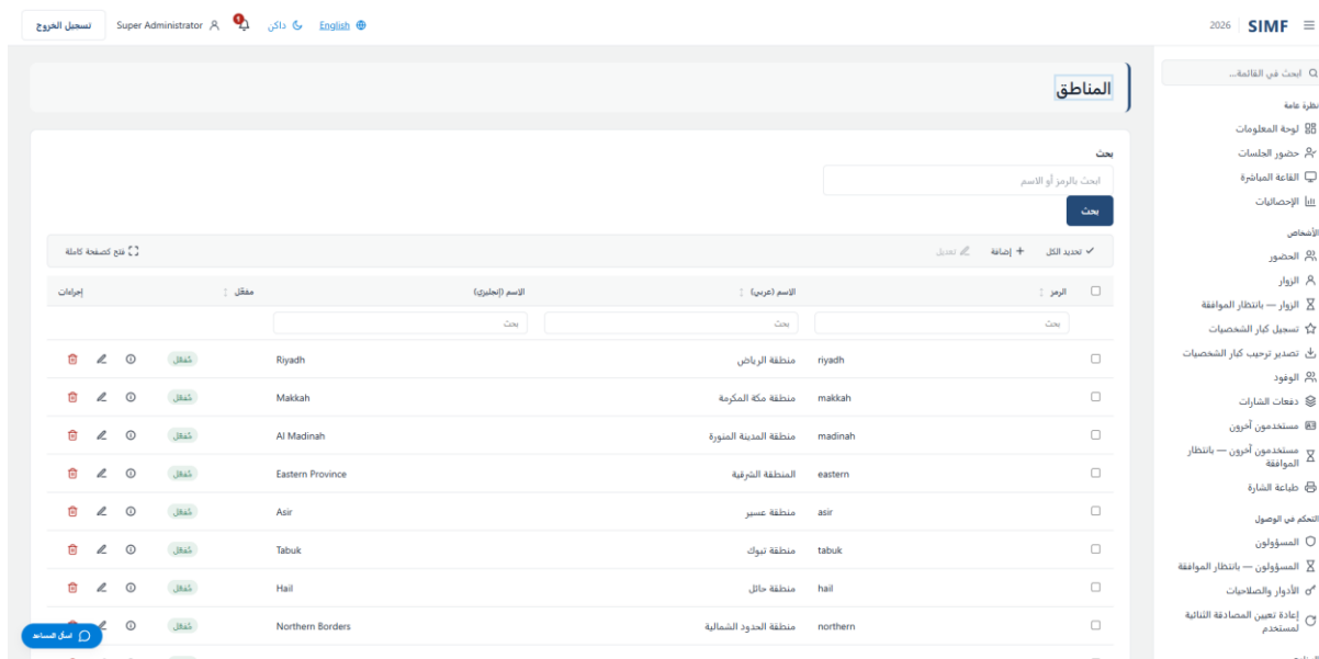
شكل 110 — المناطق — /admin/regions
