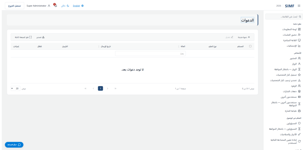
شكل 99 — الدعوات — /admin/invitations
