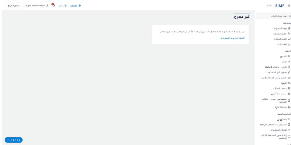
شكل 145 — /not-permitted
