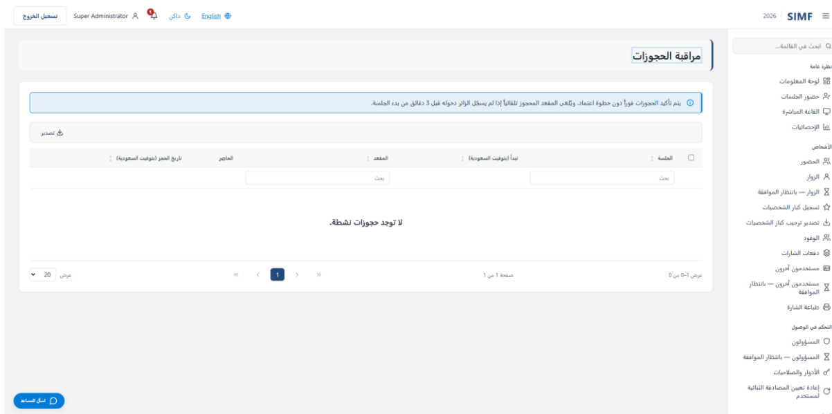
شكل 74 — الحجوزات — /admin/bookings
