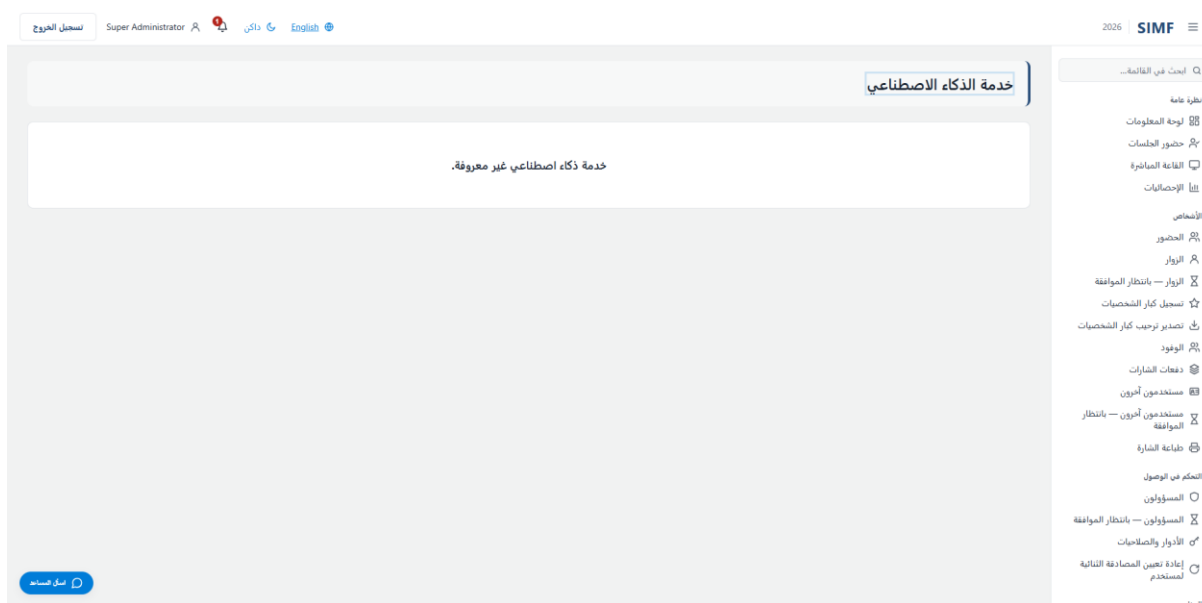
شكل 137 — /admin/ai/services/{Feature}
