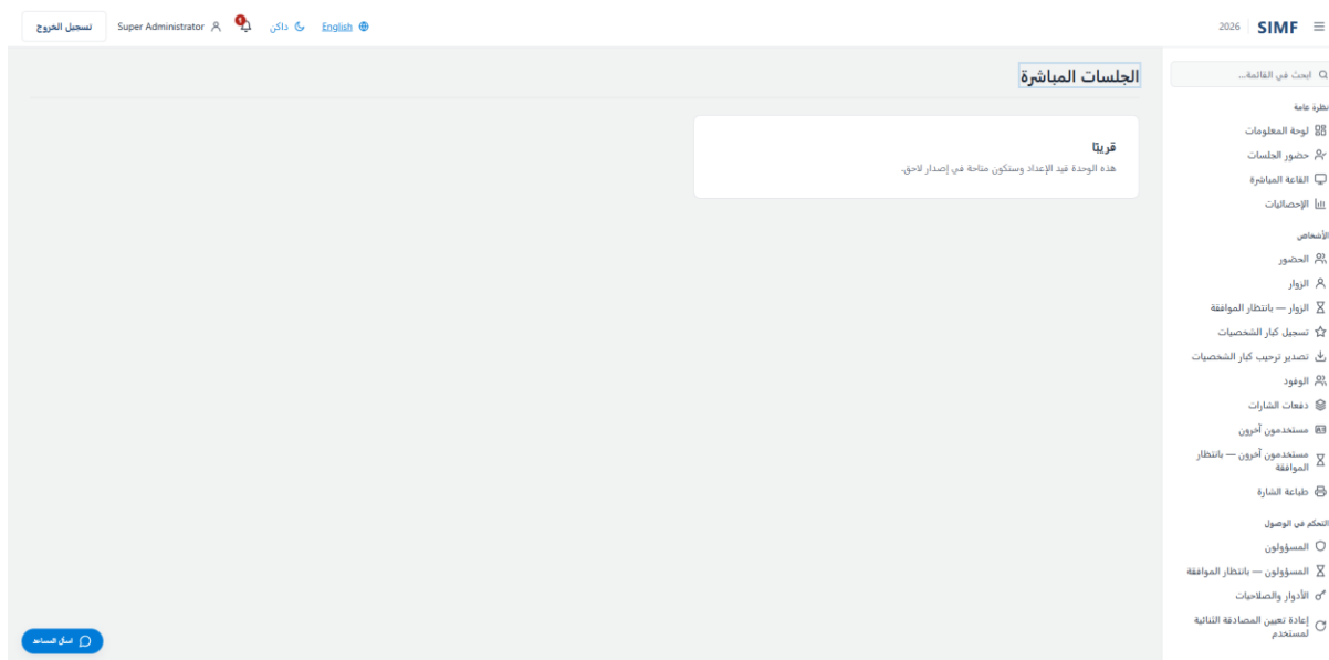
شكل 143 — /m/{Module}
