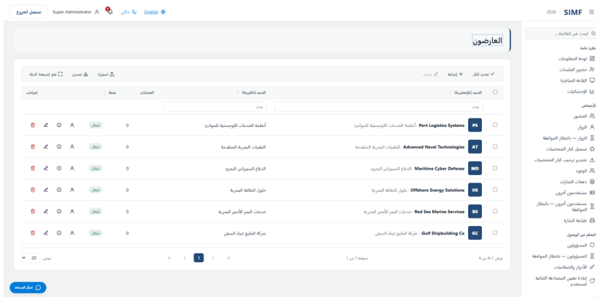
شكل 80 — العارضون — /admin/exhibitors
