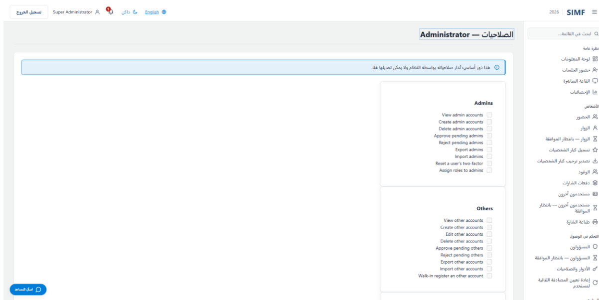
شكل 139 — /admin/roles/{RoleId:guid}/permissions
