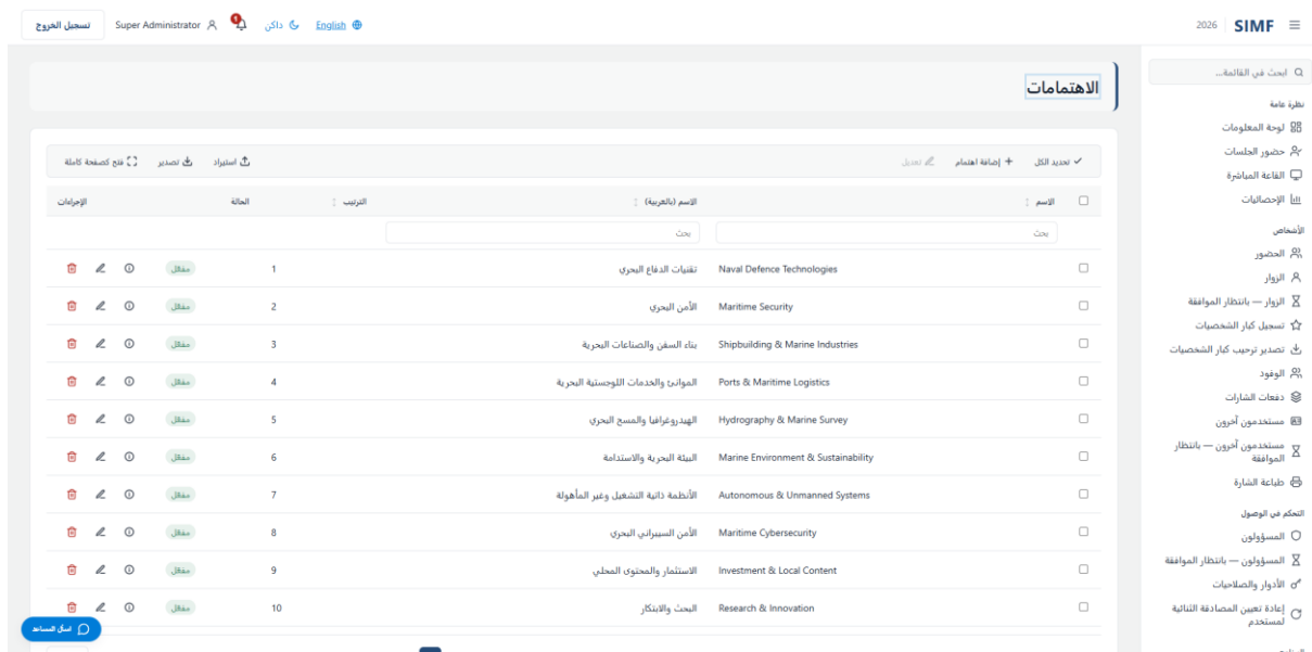
شكل 107 — الاهتمامات — /admin/interests
