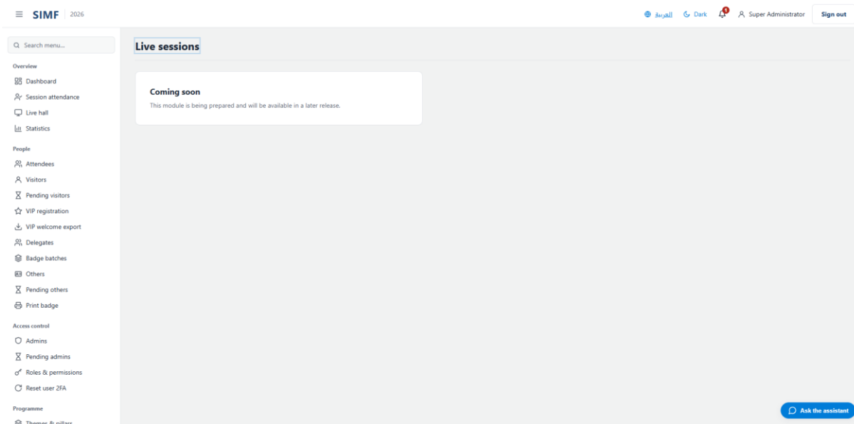
Figure 143 — /m/{Module}
