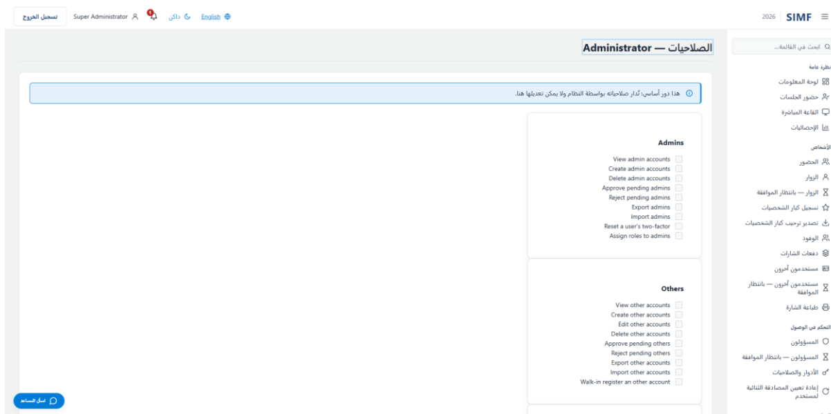
شكل 170 — /admin/roles/{RoleId:guid}/permissions
