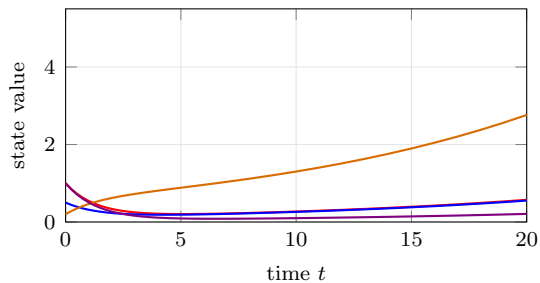
(d) x_0 = (1.0, 0.5, 0.2, 1.0)
